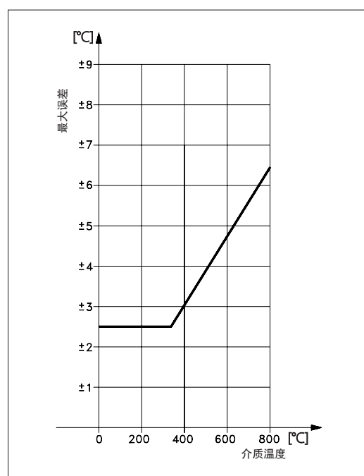
NiCr-Ni 和 Fe-CuNi
