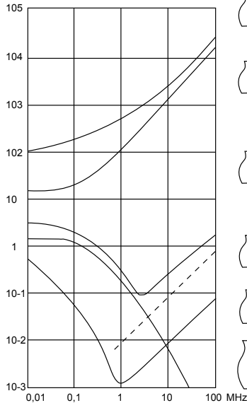
传输阻抗 Z_t \text{m}\Omega/\text{m}
