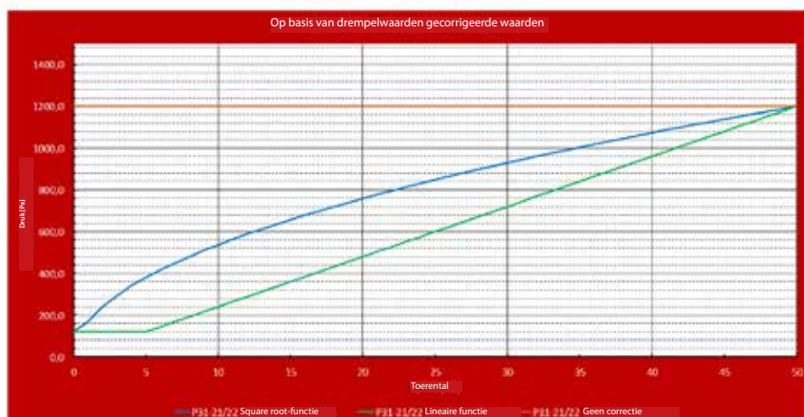
Instellingen druk-/snelheidscurve
