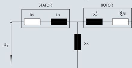
Ækvivalentkredsløb på en TPIM
