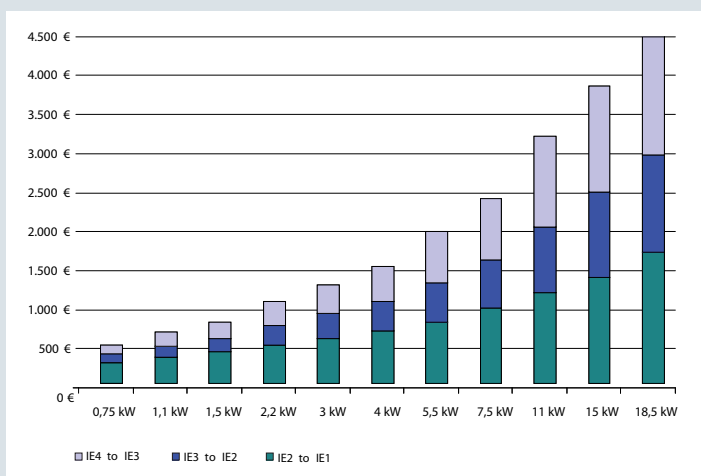
Fordelen ved omkostninger til energi for en IE motor i forhold til en IE motor i den efterfølgende bedre klasse.
