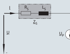
Ækvivalentkredsløb på en PMSM
