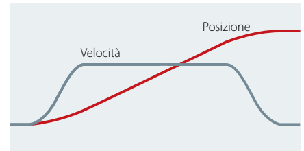
Fig. 2. Profilo del movimento con rampe S
