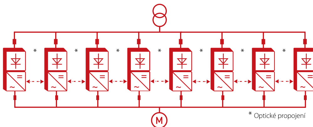
Příklad konfigurace VACON® DriveSync.
