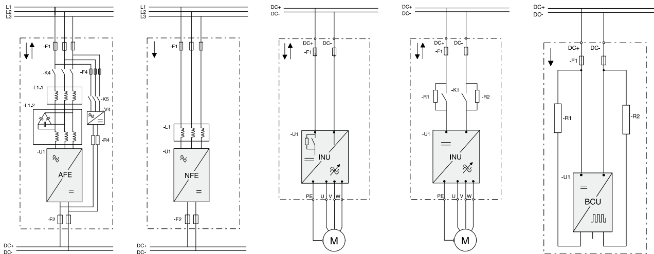
Aktives Front-End
