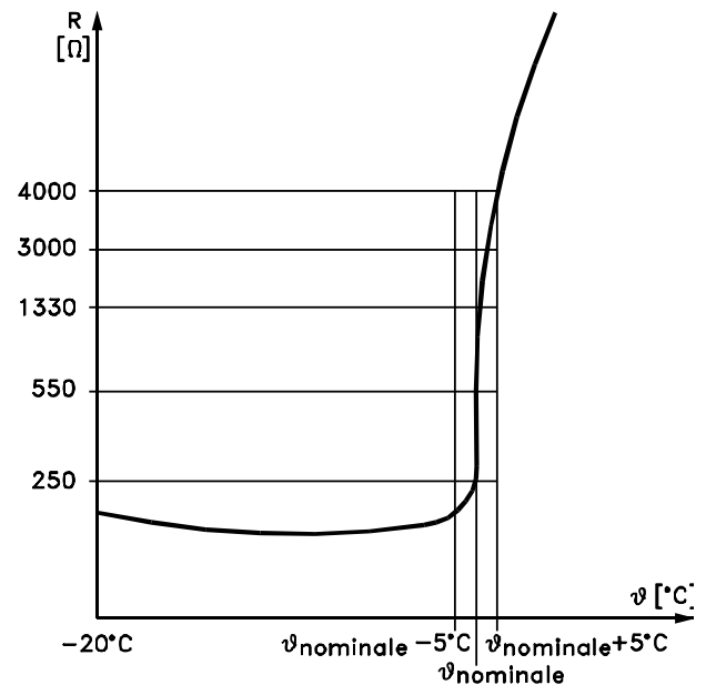
175HA183.10 Disegno 3.11 Profilo PTC
