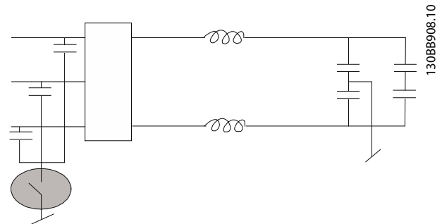
Disegno 3.42 Filtro RFI
