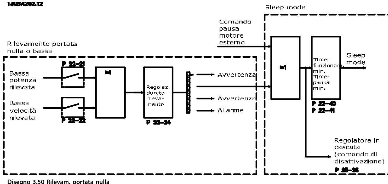
Disegno 3.50 Rilevam. portata nulla
