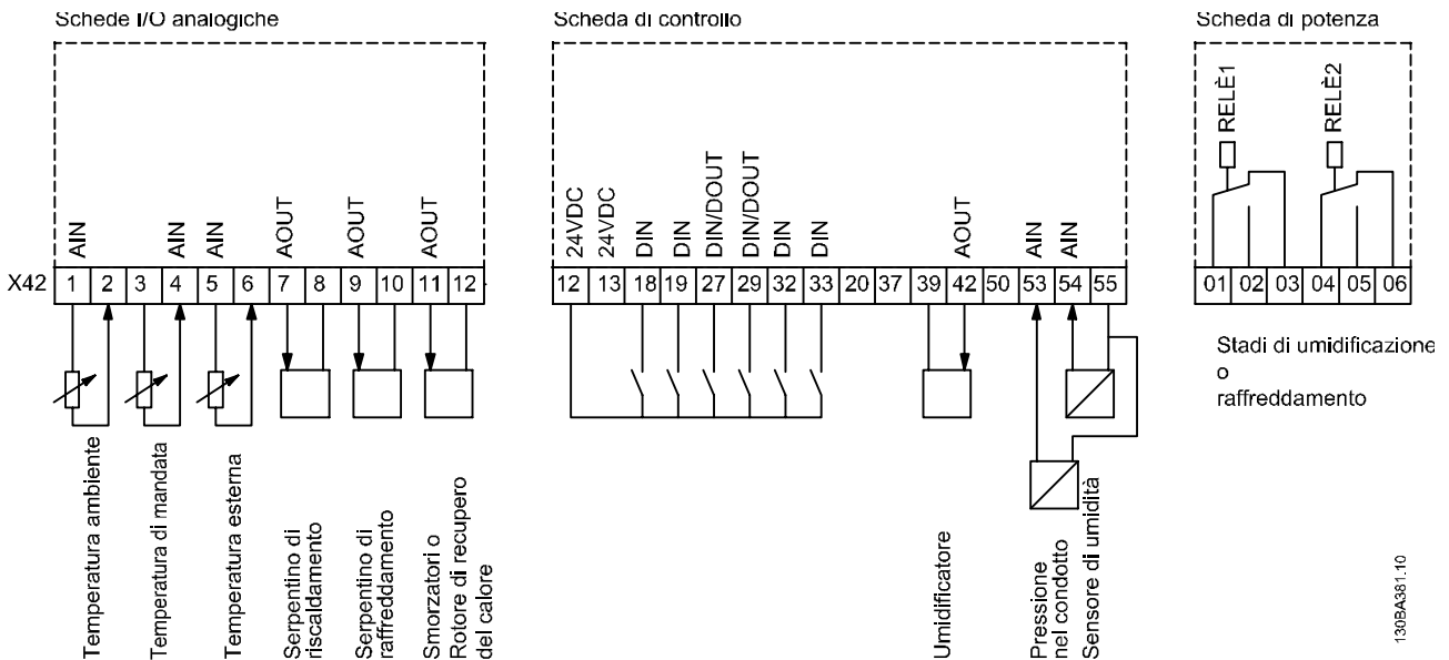
Disegno 3.83 Opzione I/O anal. MCB 109
