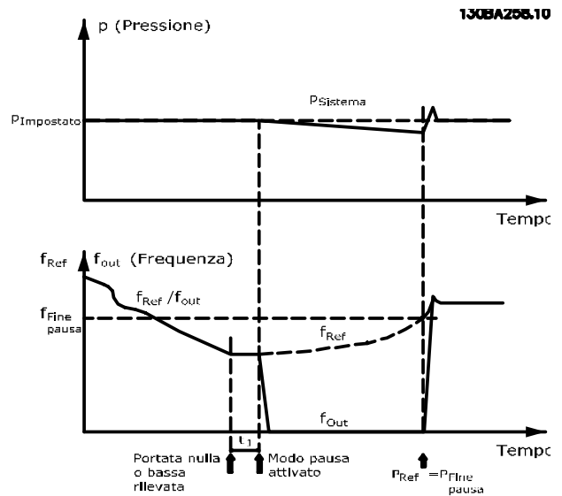
Disegno 3.54 Sistema di sovralimentazione
