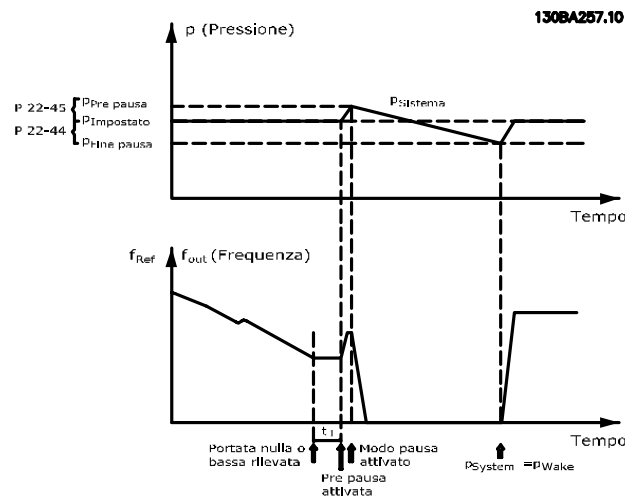
Disegno 3.52 Sistema di sovralimentazione
