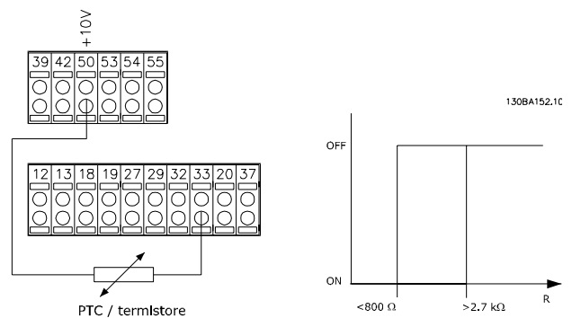
Disegno 3.12 Collegamento termistore PTC - ingresso digitale
