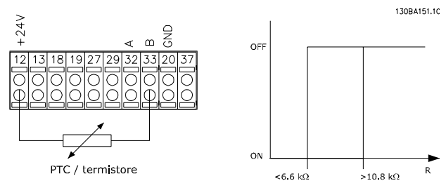
Disegno 3.15 Collegamento termistore
