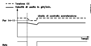
Disegno 3.39 Backup dell'energia cinetica, guasto di rete breve
