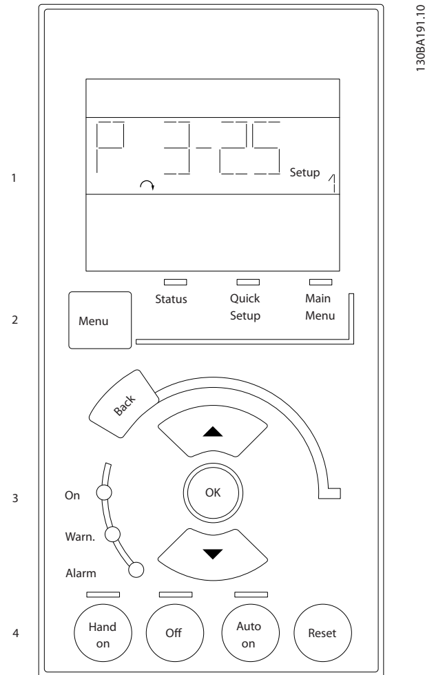
Disegno 2.13 LCP numerico (NLCP)
