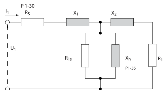
Disegno 3.4 Grafico equivalente per un motore asincrono
