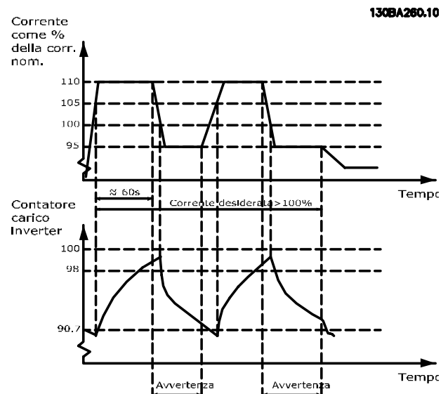
Disegno 3.43 Corrente di uscita nella corrente di sovraccarico
