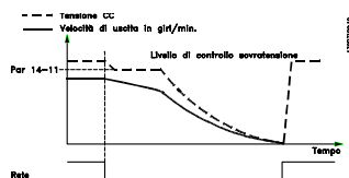
Disegno 3.40 Backup dell'energia cinetica, guasto di rete prolungato
