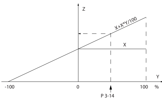
Disegno 3.19 Riferimento corrente
