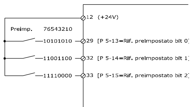
Disegno 3.16 Schema di riferimento preimpostato
