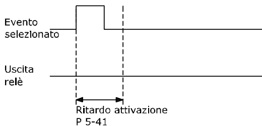
Disegno 3.25 Ritardo attivato, relè
