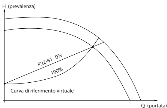
Disegno 3.57 Appross. lineare-quadratica
