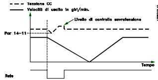
Disegno 3.37 Rampa di decelerazione controllata - guasto di rete breve
