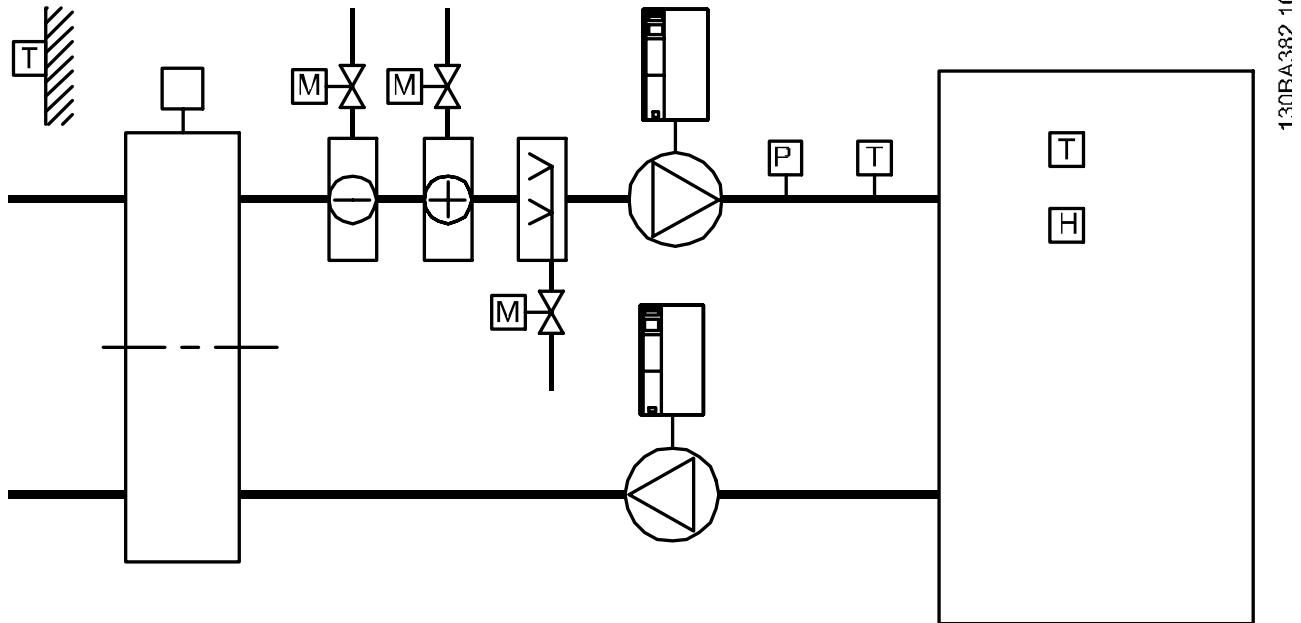
Disegno 3.82 Opzione I/O anal. MCB 109
