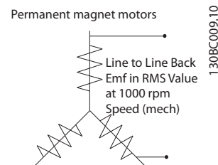
Disegno 3.7 Definizioni dei parametri macchina della forza c.e.m di motori PM
