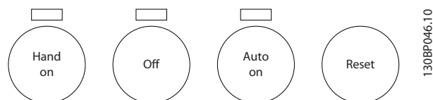
Disegno 2.17 Tasti di comando dell'LCP numerico (NLCP)
