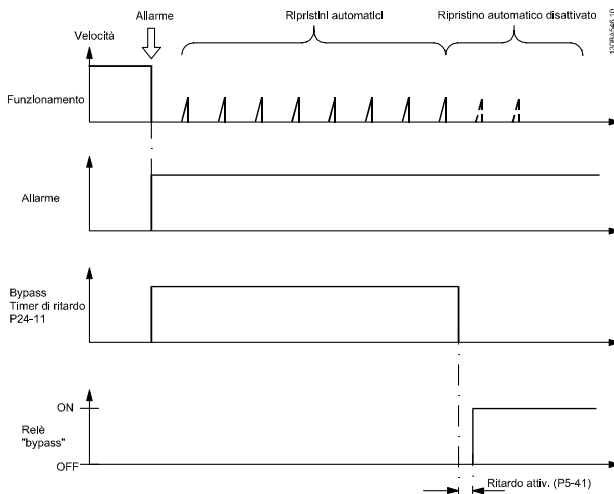
Disegno 3.66 Bypass inverter
