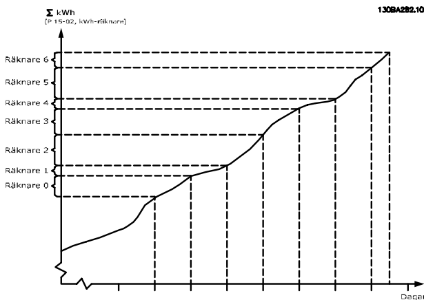
Bild 3.59 Energilogg, diagram
