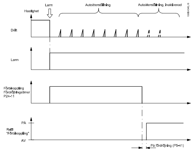
Bild 3.64 Förbikoppling
