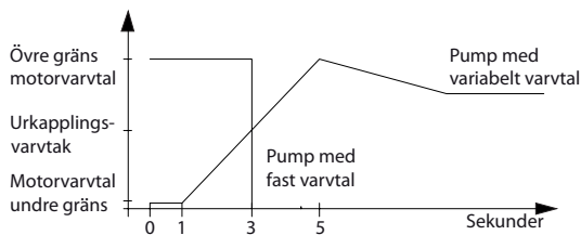
Bild 3.77 Urkopplingströskel
