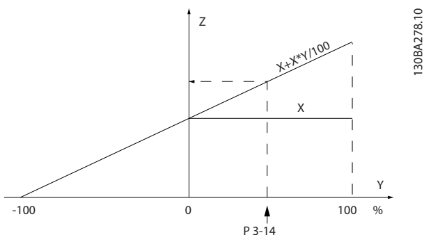
Bild 3.14 Faktisk referens
