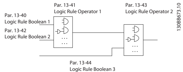
Bild 3.31 Logiska regler
