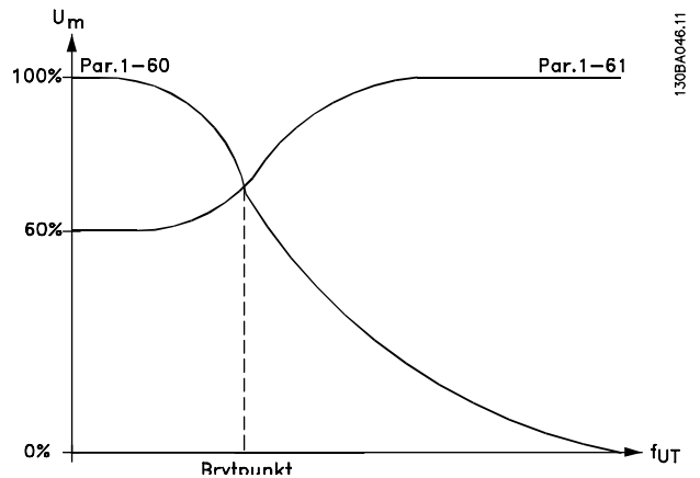
Bild 3.9 Lastkompensation för lågt varvtal
