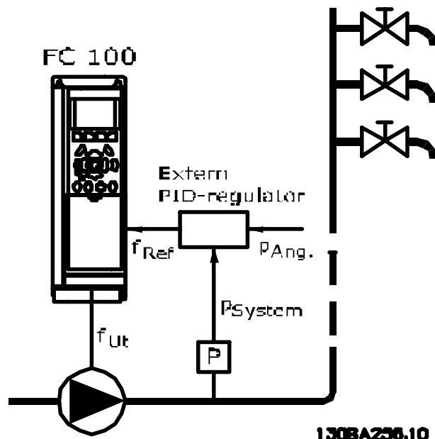
Bild 3.50 Stegringsystem
