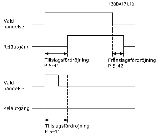
Bild 3.20 Till-fördr., relä
