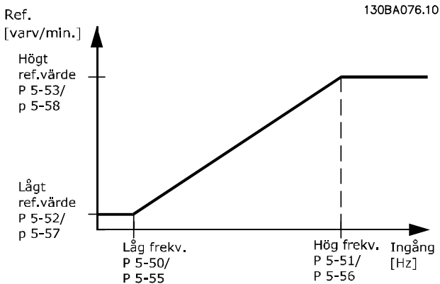
Bild 3.22 Pulsingång
