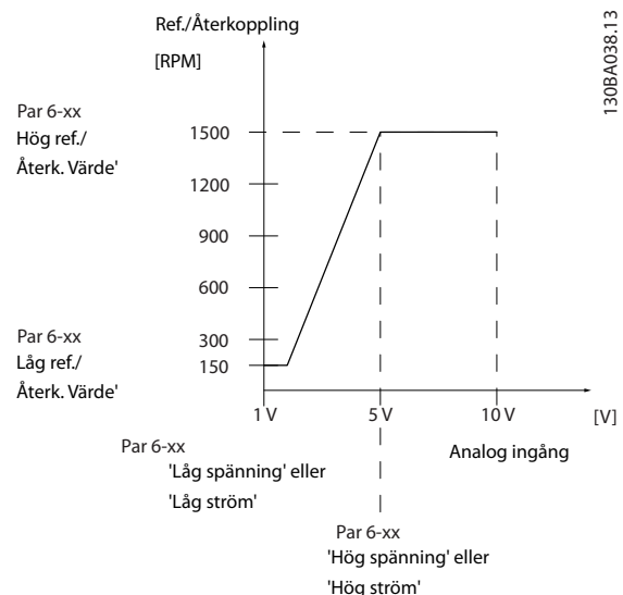
Bild 3.24 Signalavbrottsförhållanden
