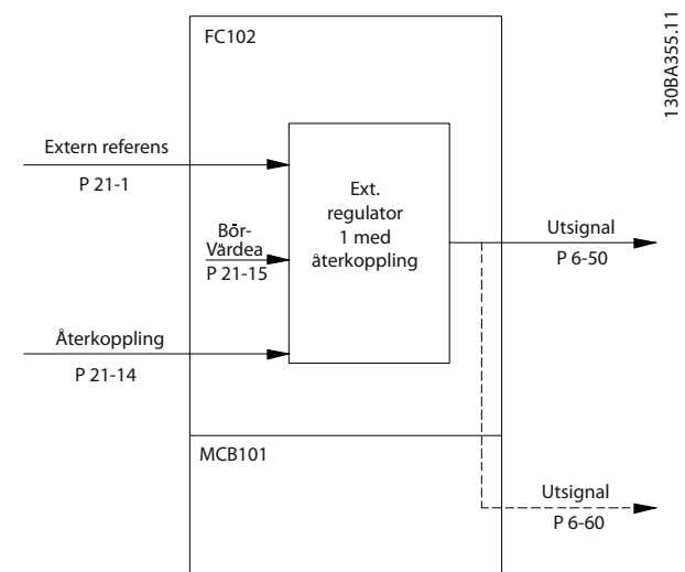
Bild 3.46 Med återkoppling 1, ref./återk.
