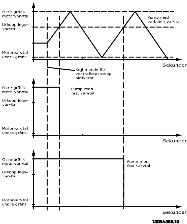
Bild 3.78 Urkopplingsvarvtal
