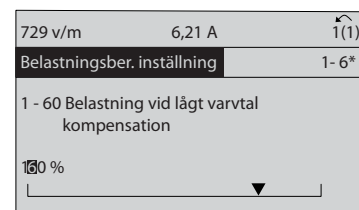
Bild 2.31 Ändra en grupp med numeriska datavärden
