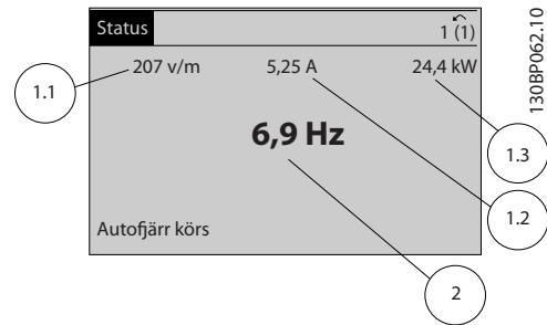
Bild 2.3 Exempel på statusdisplay II
