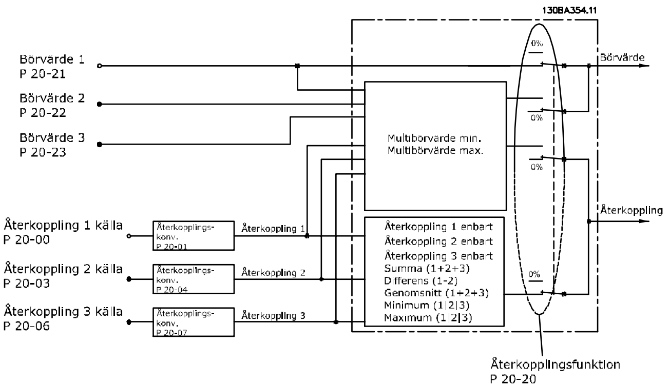
Bild 3.44 Återkoppling
