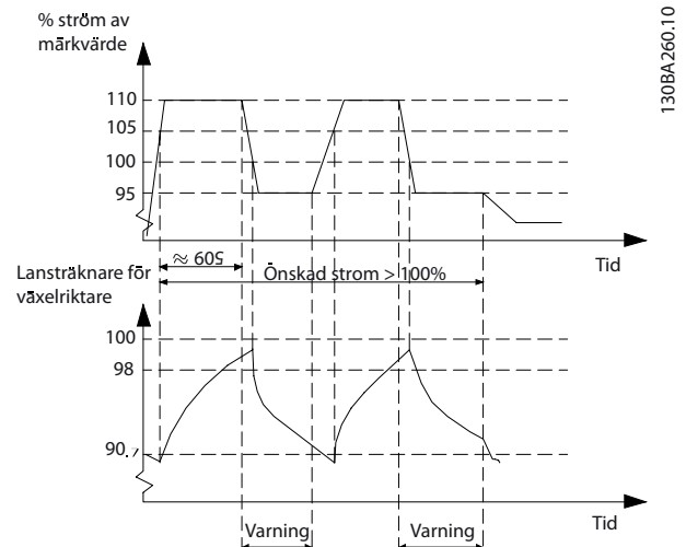
Bild 3.38 Utström vid överbelastning
