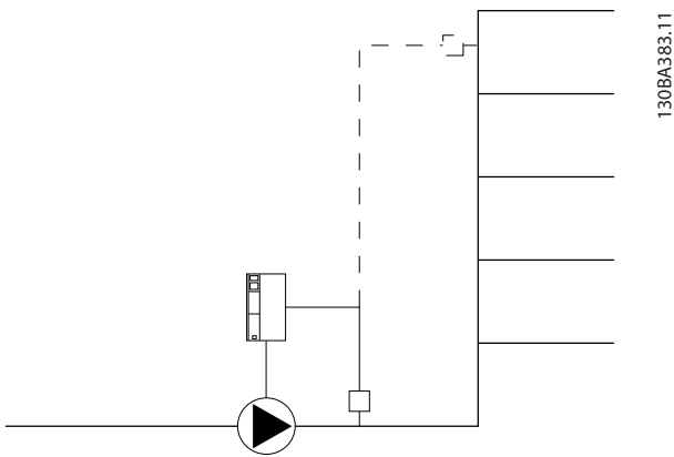
Bild 3.52 Flödeskompensation
