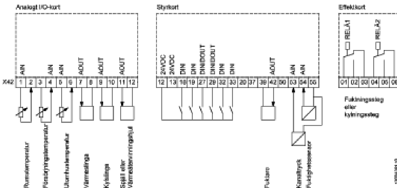
Bild 3.81 Analogt I/O-tillval MCB 109
