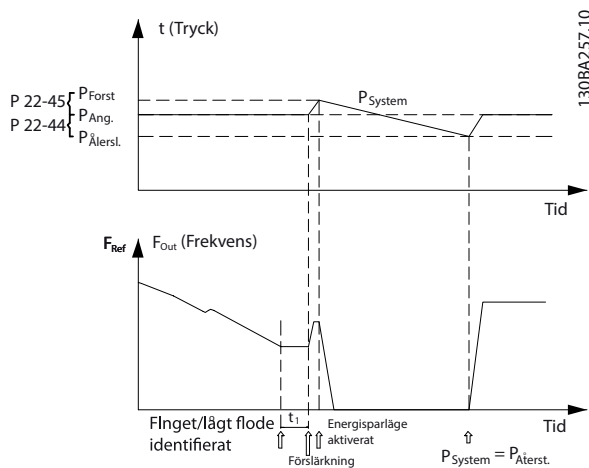
Bild 3.49 Stegringsystem
