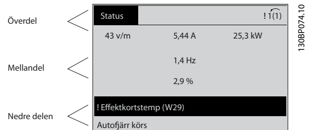
Bild 2.5 Displayavsnitt
