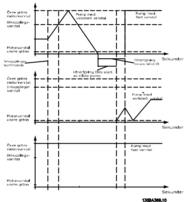
Bild 3.79 Inkopplingsläge vid alternering
