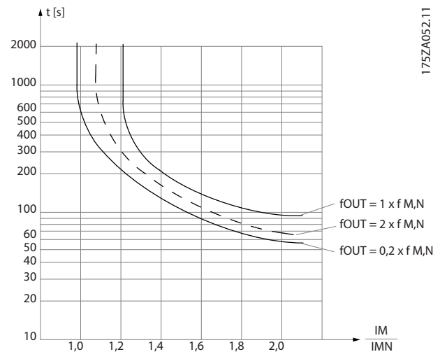
Bild 3.10 Termiskt motorskydd
