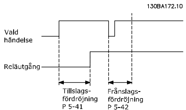
Bild 3.21 Från-fördr., relä
