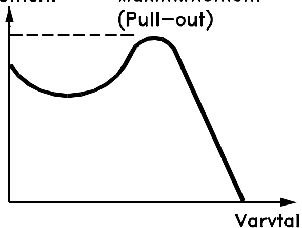
DANFOSS 175ZA078.10 Bild 1.1 Startmoment
