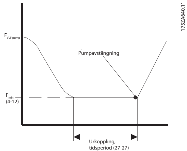
Bild 3.73 Tid för urkopplingsfunktion
