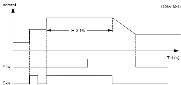
Bild 3.18 Rampfördröjning, fall 2
