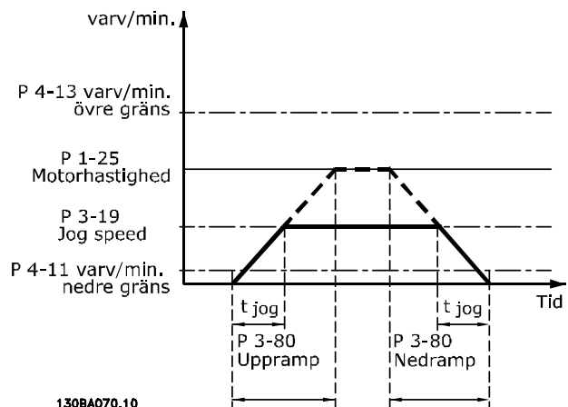
130BA070.10 Bild 3.16 Joggramptid
