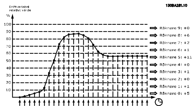
Bild 3.62 Tid och relativa värden
