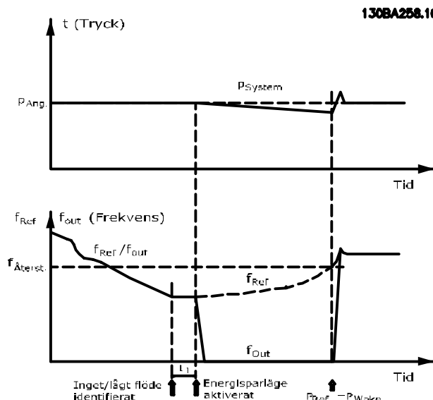
Bild 3.51 Stegringsystem
