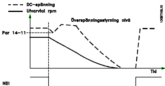
Bild 3.33 Kontrollerad nedrampning, längre nätfel. Nedrampning så länge som energin i systemet tillåter detta, sedan rullas motorn ut.
