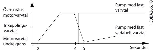
Bild 3.76 Inkopplingströskel
