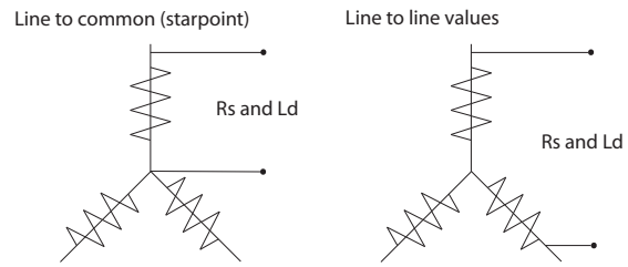
Bild 3.6 Statorlindningsinställningar
