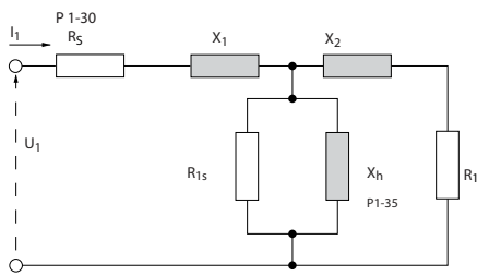
Bild 3.4 Ekvivalensdiagram för en asynkronmotor
