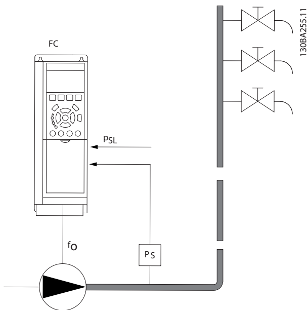
Bild 3.48 Energisparläge
