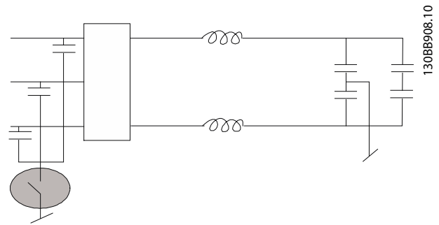
Bild 3.37 RFI-filter
