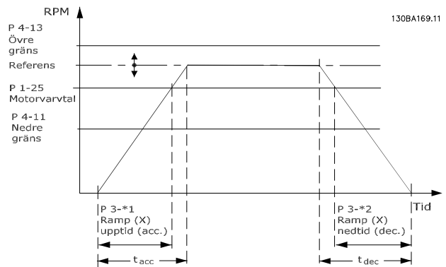
Bild 3.15 Ramp 1
