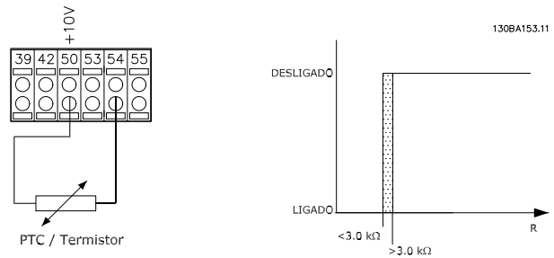
图 3.13 PTC 热敏电阻连接 - 模拟输入
