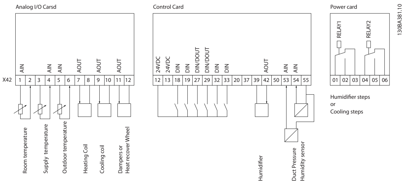
图 3.83 模拟 I/O 选项 MCB 109
