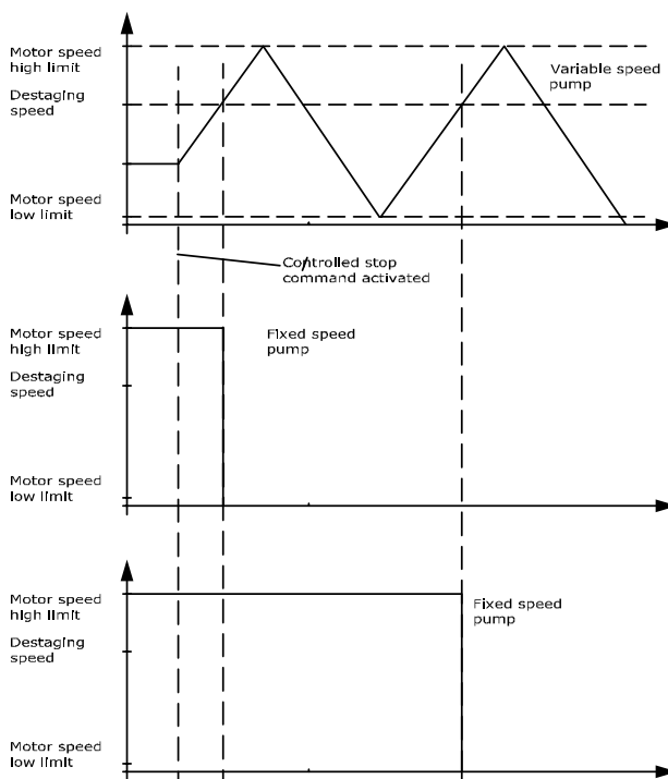
图 3.80 停止速度
