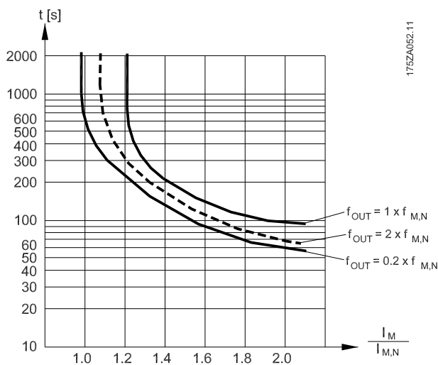
图 3.10 电动机热保护
