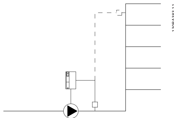
图 3.55 流量补偿
