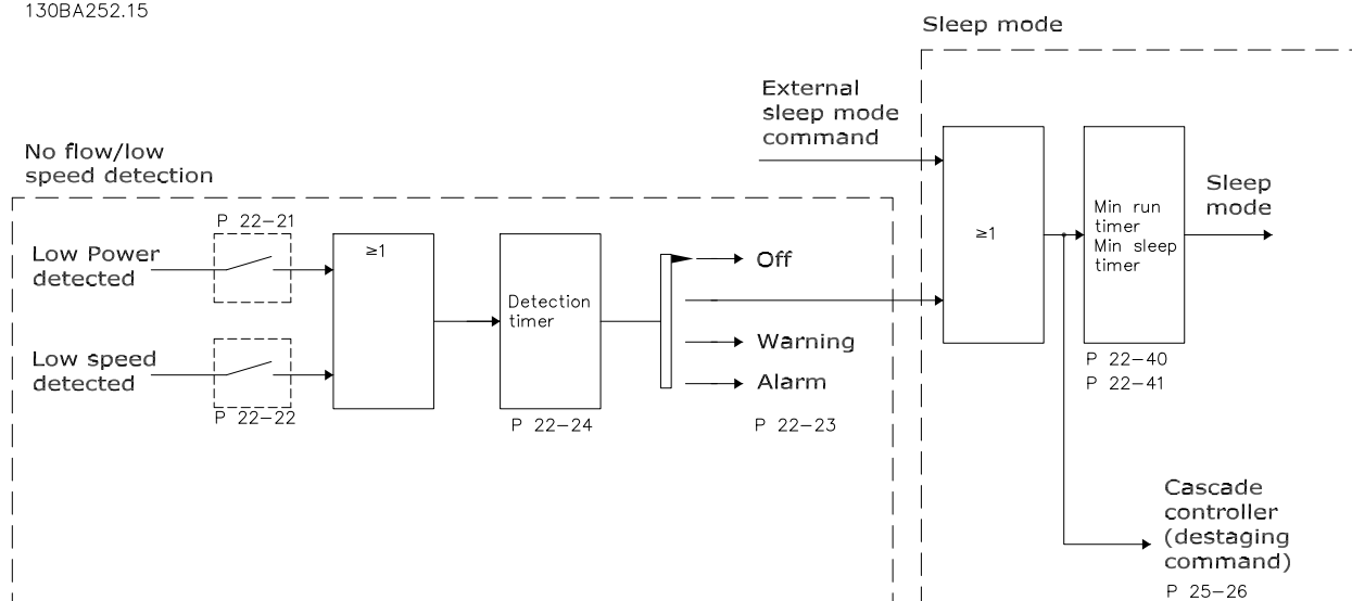
图 3.50 无流量检测
