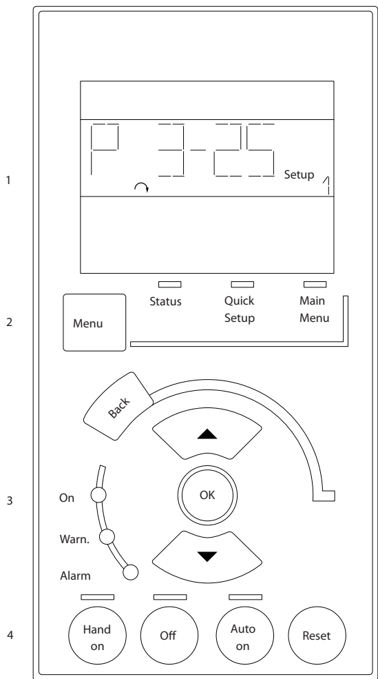
图 2.13 数字式 LCP (NLCP)
