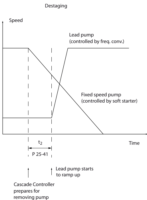
图 3.77 正在停止
