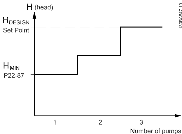
图 3.56 泵数量
