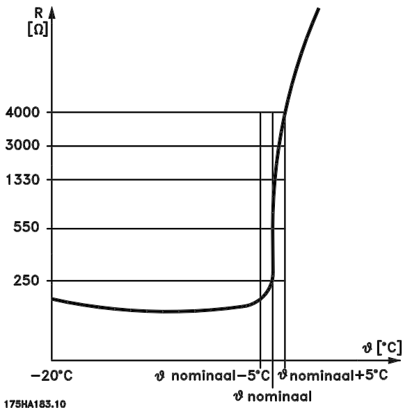
图 3.11 PTC 协议
