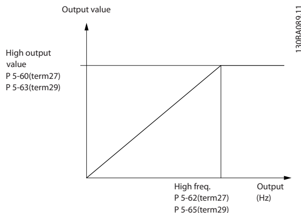
图 3.28 脉冲输出
