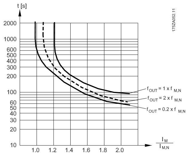
图 3.14 ETR 协议
