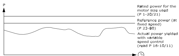
图 3.65 变速控制
