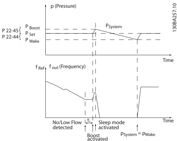
图 3.52 放大系统
