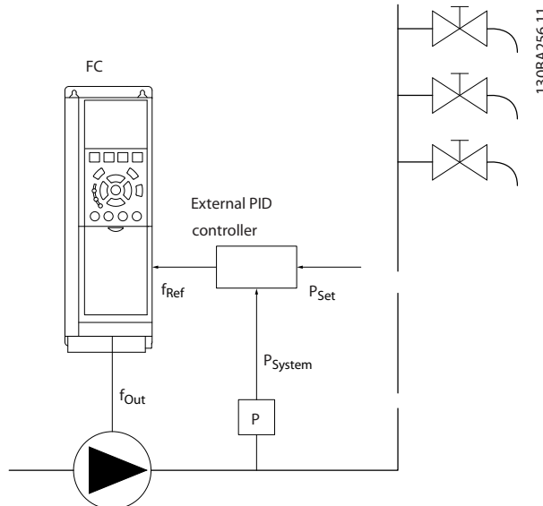
图 3.53 放大系统
