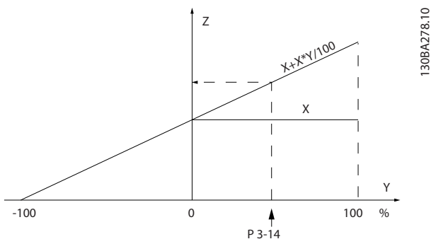
图 3.19 实际参考值
