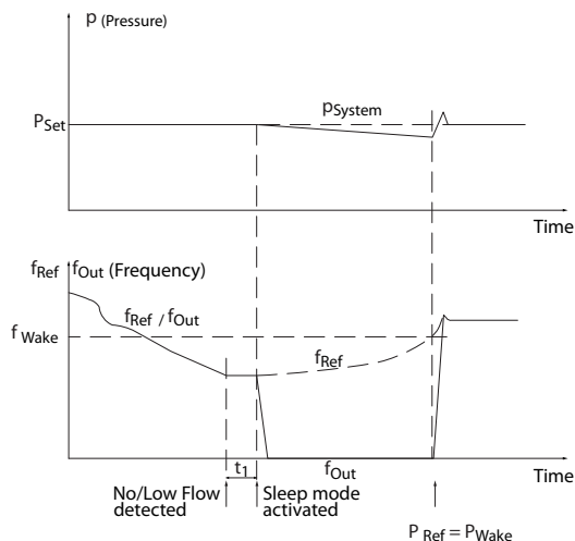
图 3.54 放大系统
