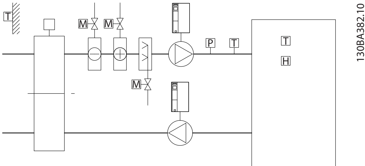
图 3.82 模拟 I/O 选项 MCB 109
