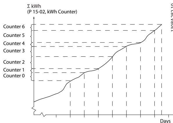
图 3.62 能量记录图
