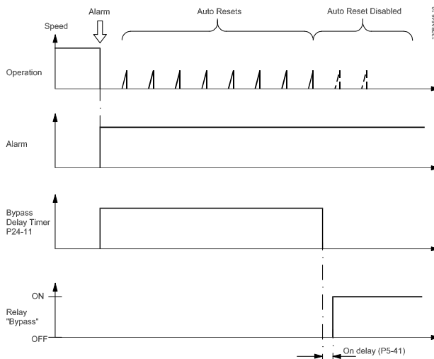
图 3.66 变频器旁路
