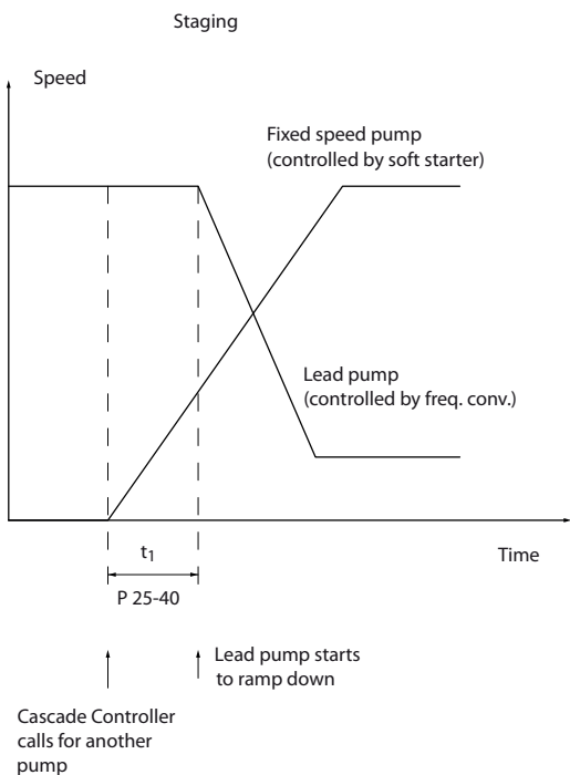
图 3.76 正在切入
