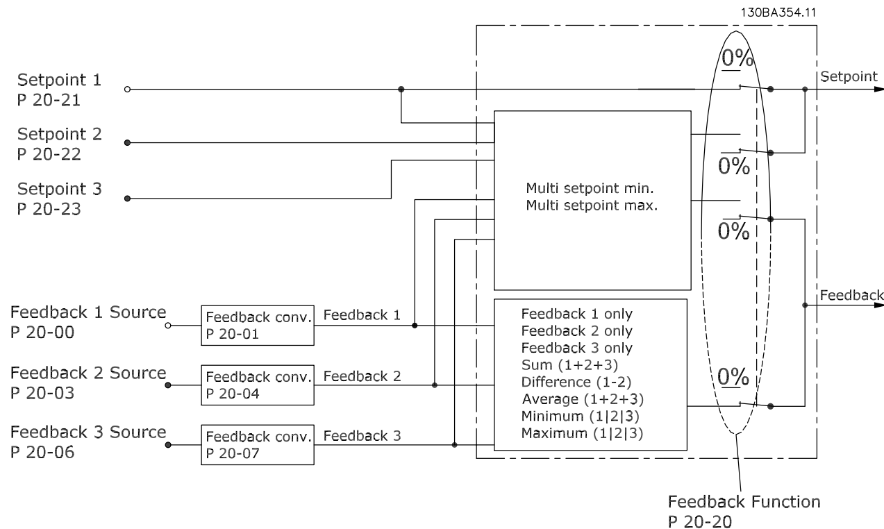
图 3.47 反馈
