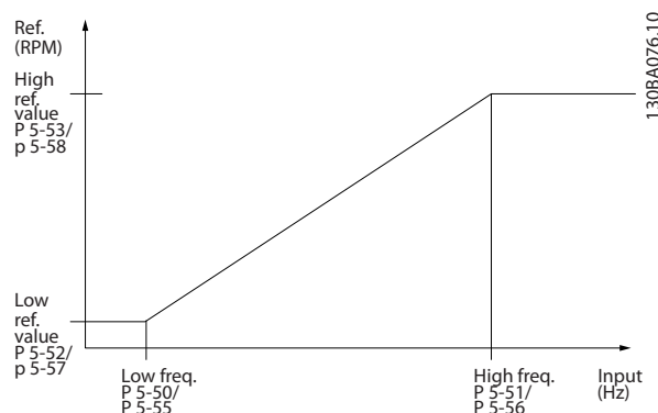
图 3.27 脉冲输入
