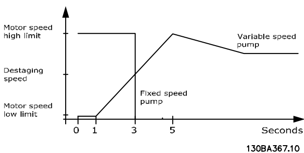
图 3.79 停止阈值
