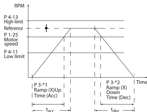
图 3.20 加减速 1
