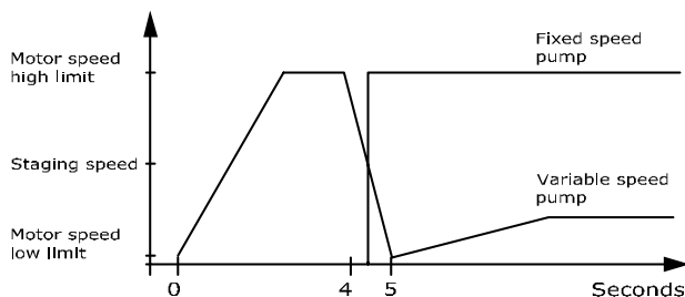
图 3.78 切入阈值
