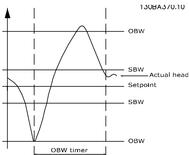
图 3.74 OBW 时间
