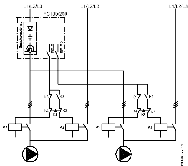
Ilustracija 8.8 Shema ožičenja izmeničnega delovanja vodilne črpalke
