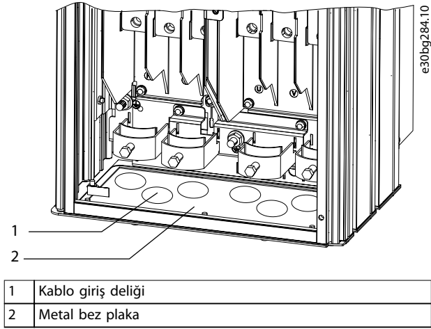
Çizim 4.4 Sac Metal Bez Plakadaki Kablo Açıklıkları
