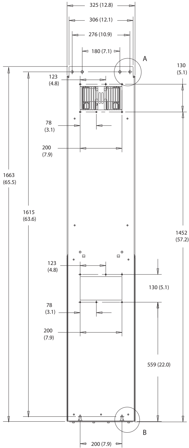
Çizim 10.26 D6h'nin Arkadan Görünümü
