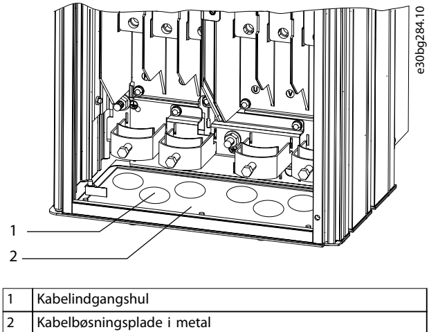
Illustration 4.4 Kabelåbninger i kabelbøsningsplade i metal
