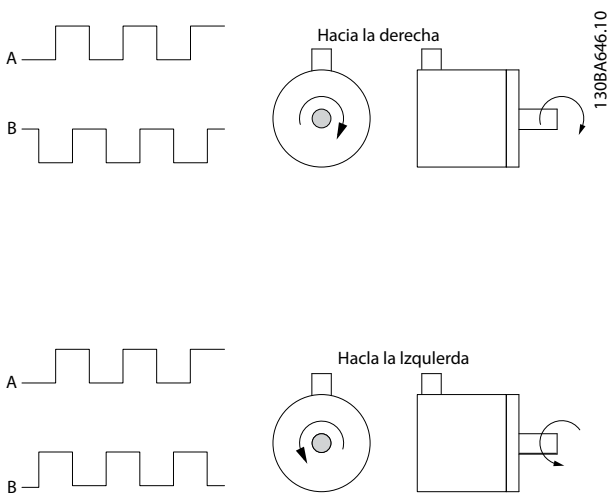
Ilustración 8.6 Determinar la dirección del encoder
