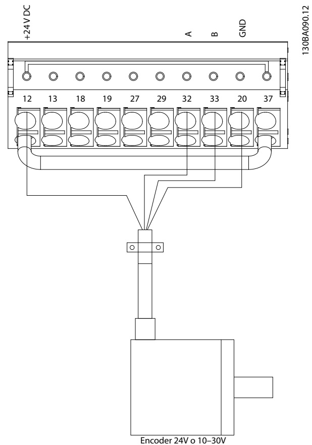
Disegno 8.7 Configurazione del filo per l'encoder
