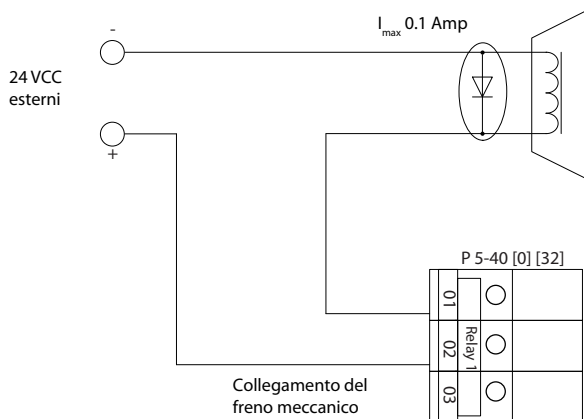
Disegno 8.8 Configurazione dei fili per il limite di coppia e di arresto
