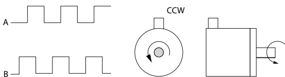
Disegno 8.6 Individuazione della direzione dell'encoder
