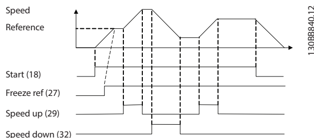
Slika 8.4 Ubrzanje/usporenje
