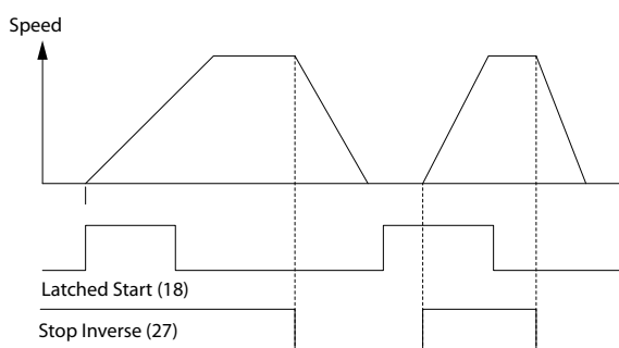
Slika 8.3 Pulsni start/inverzno zaustavljanje
