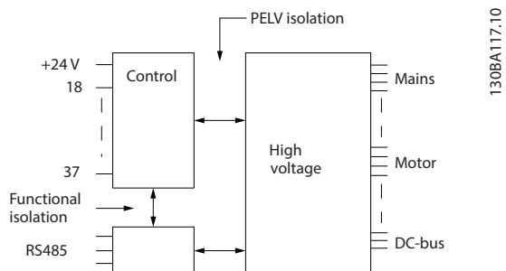
Slika 10.1 PELV izolacija
