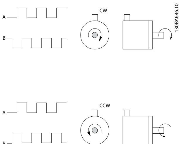
Slika 8.6 Određivanje smisla vrtnje enkodera
