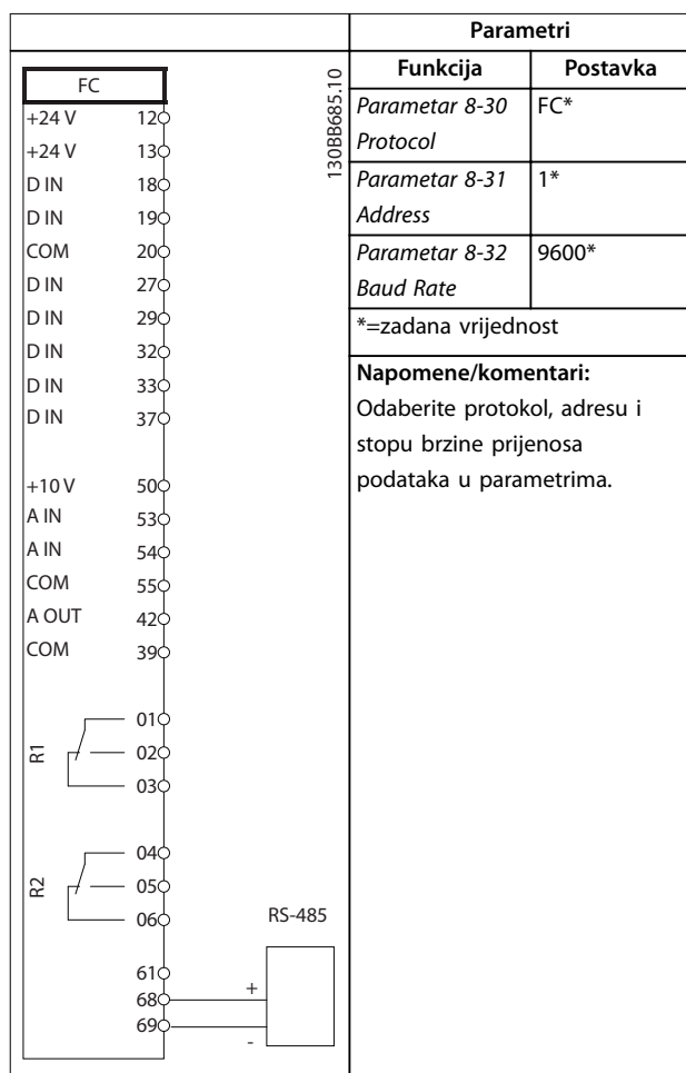
Tablica 8.11 Konfiguracija ožičenja za RS485 mrežni priključak
