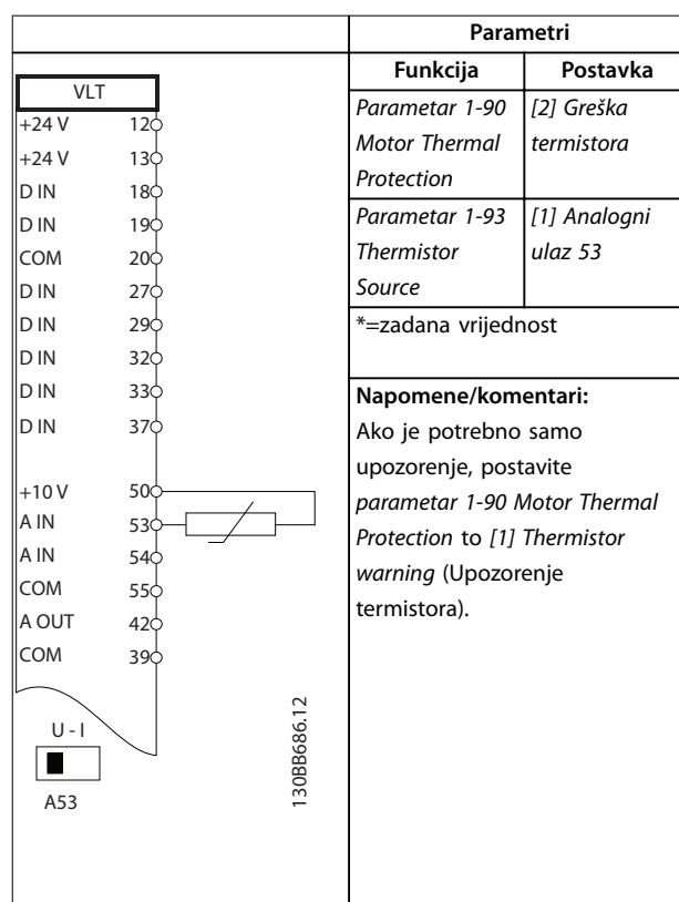
Tablica 8.12 Konfiguracija ožičenja za termistor motora
