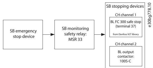
Illustration 5.6 Sikkerhedsrelateret blokdiagram
