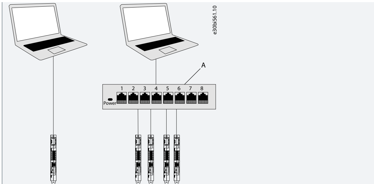
Abbildung 17: Anschluss an den PC
