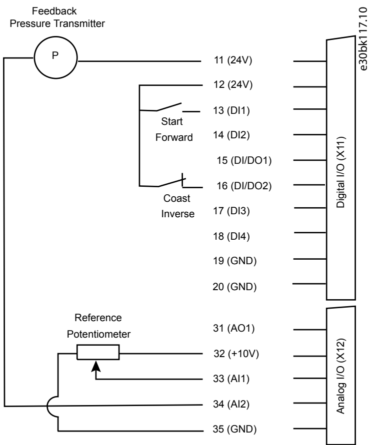
Abbildung 46: Beispiel für einen Schaltplan – Prozessregelung mit Basis-E/A
