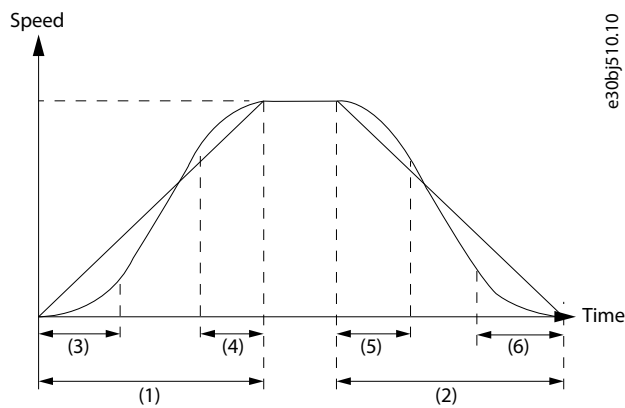
Abbildung 60: Drehzahlrampen
