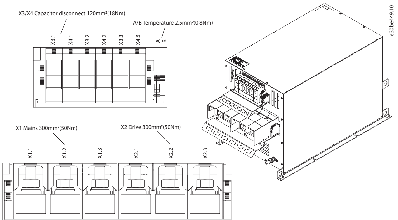
Abbildung 7.33 IP20 X8-V3 Externer Lüfter, Klemmenbezeichnung und 3D-Ansicht
