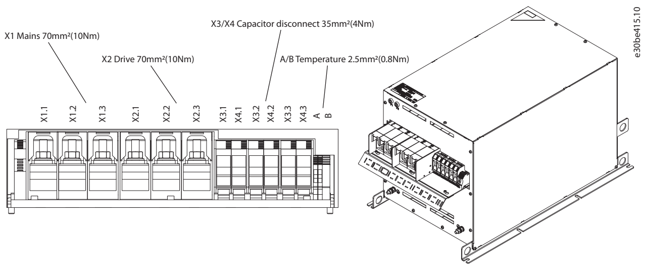
Abbildung 7.25 IP20 X6-V3 Externer Lüfter, Klemmenbezeichnung und 3D-Ansicht
