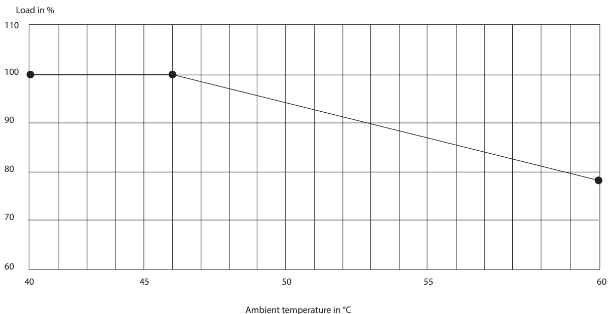
Abbildung 7.1 Temperatur – Leistungsreduzierungskurve
