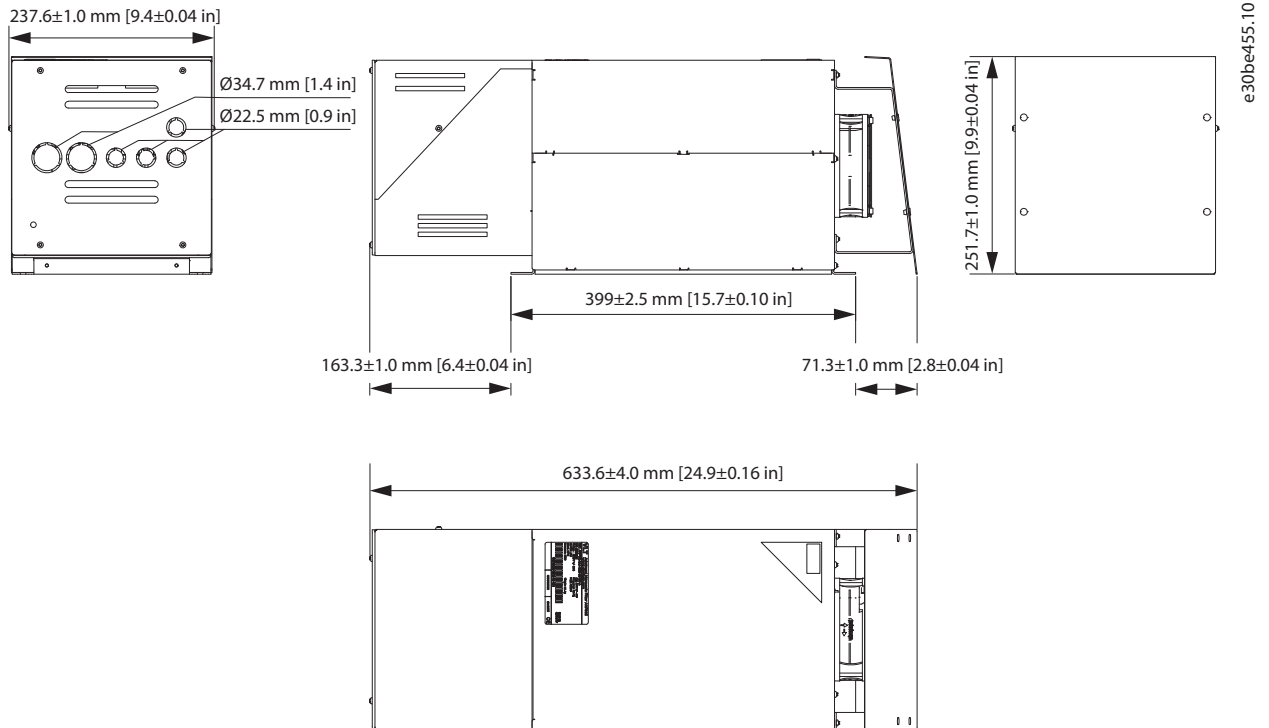
Abbildung 7.36 IP21 X2-V3 interner und externer Lüfter
