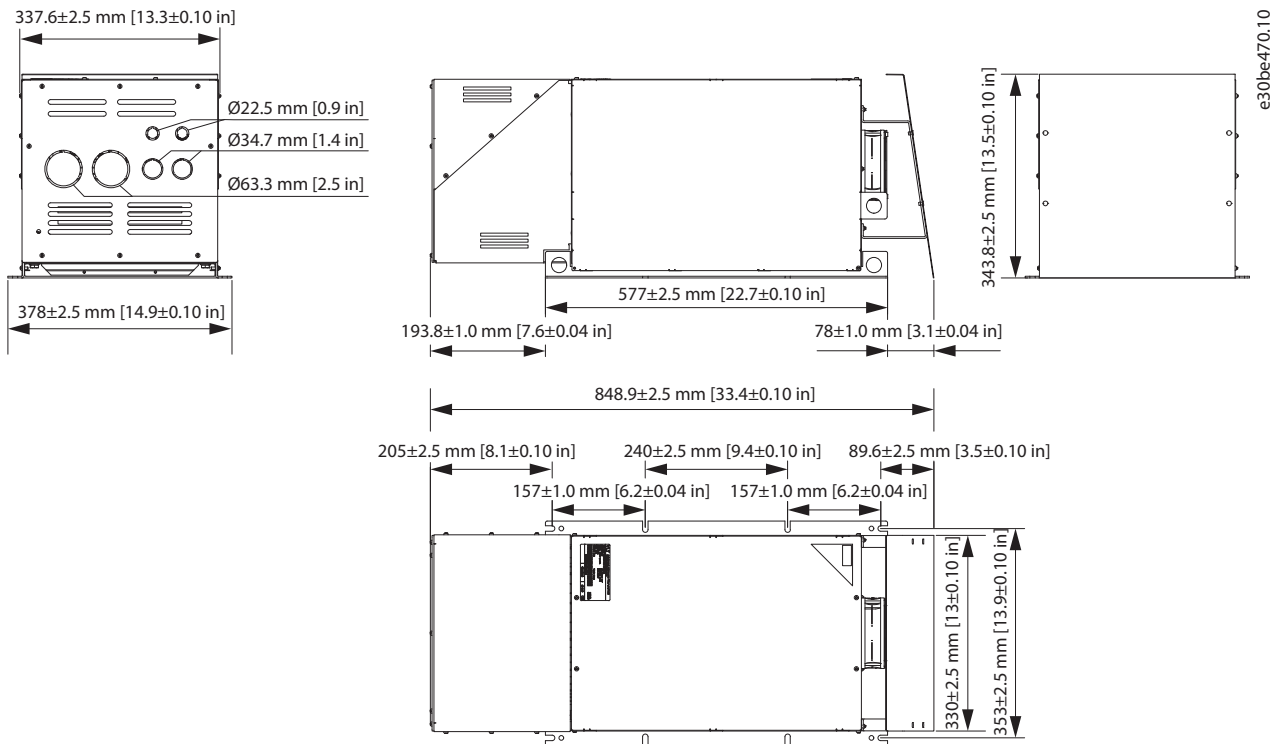
Abbildung 7.40 IP21 X4-V3 interner und externer Lüfter
