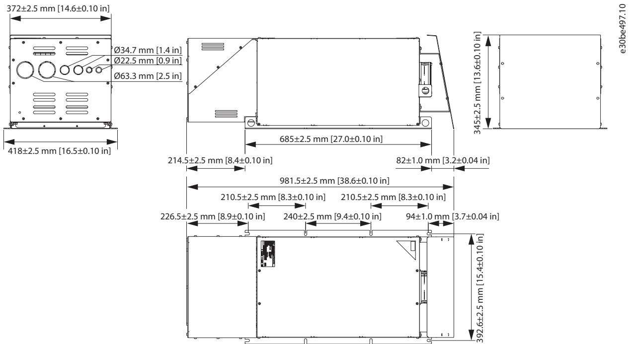
Abbildung 7.42 IP21 X5-V3 interner und externer Lüfter
