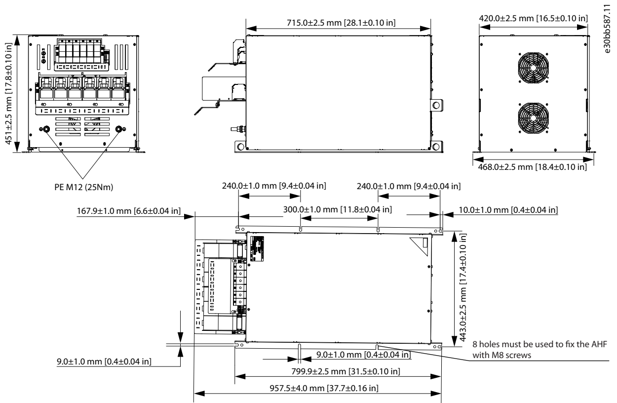
Abbildung 7.26 IP20 X7-V3 Interner Lüfter
