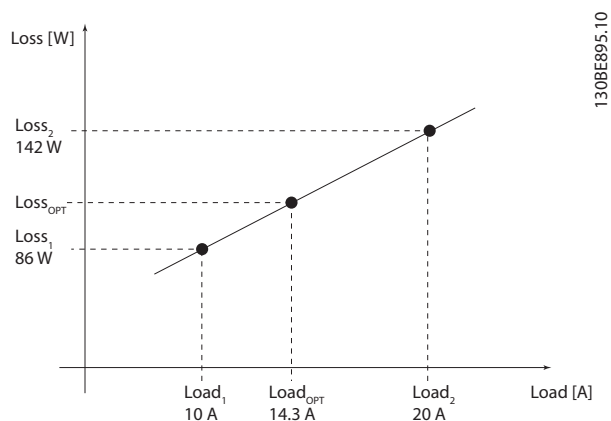
Abbildung 9.5 Bestimmen der Verlustleistung mit 2-dimensionaler Interpolation
