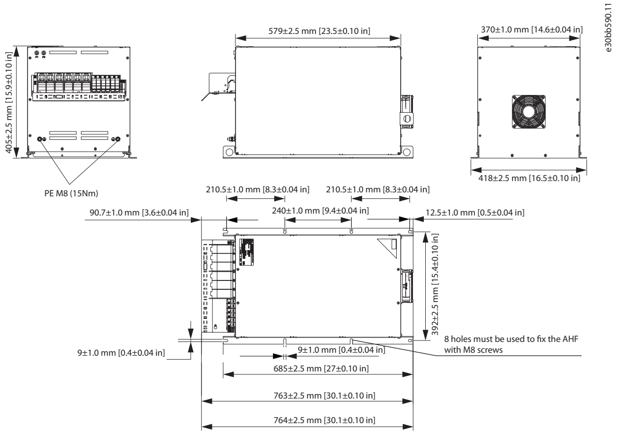
Abbildung 7.24 IP20 X6-V3 Externer Lüfter
