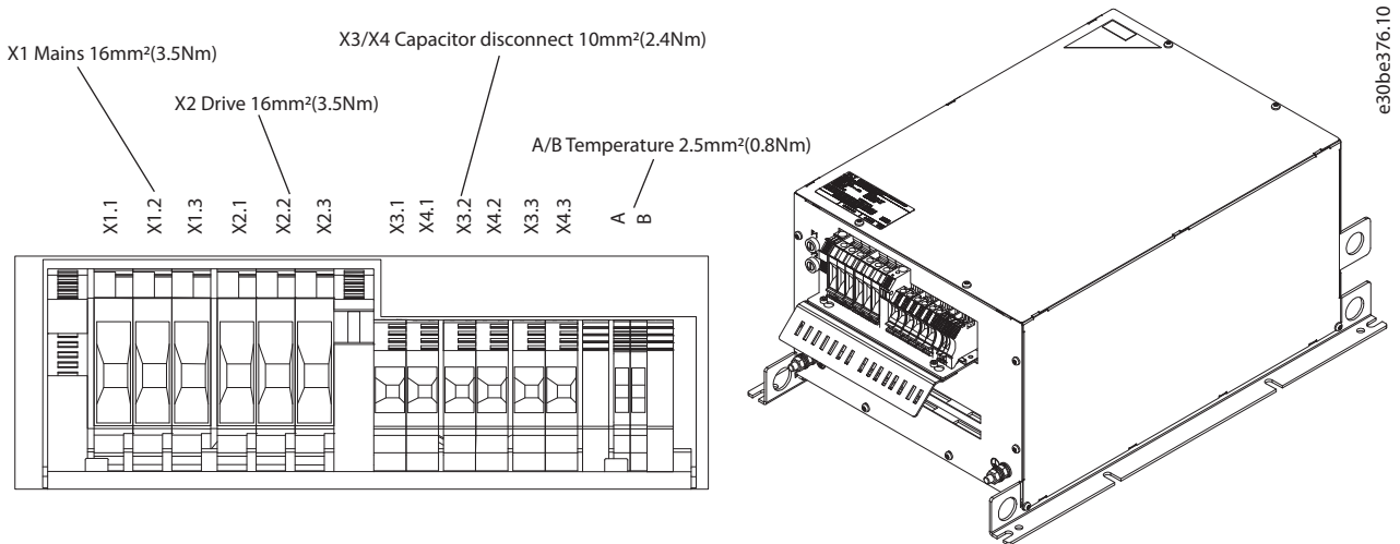
Abbildung 7.13 IP20 X3-V3 Externer Lüfter, Klemmenbezeichnung und 3D-Ansicht
