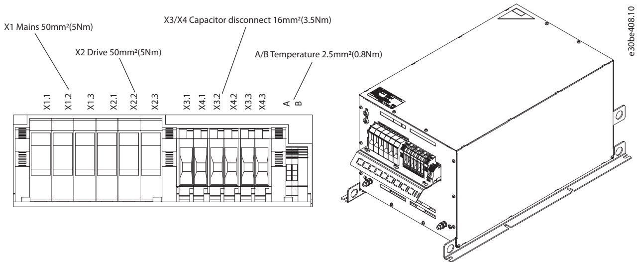
Abbildung 7.19 IP20 X5-V3 Interner Lüfter, Klemmenbezeichnung und 3D-Ansicht
