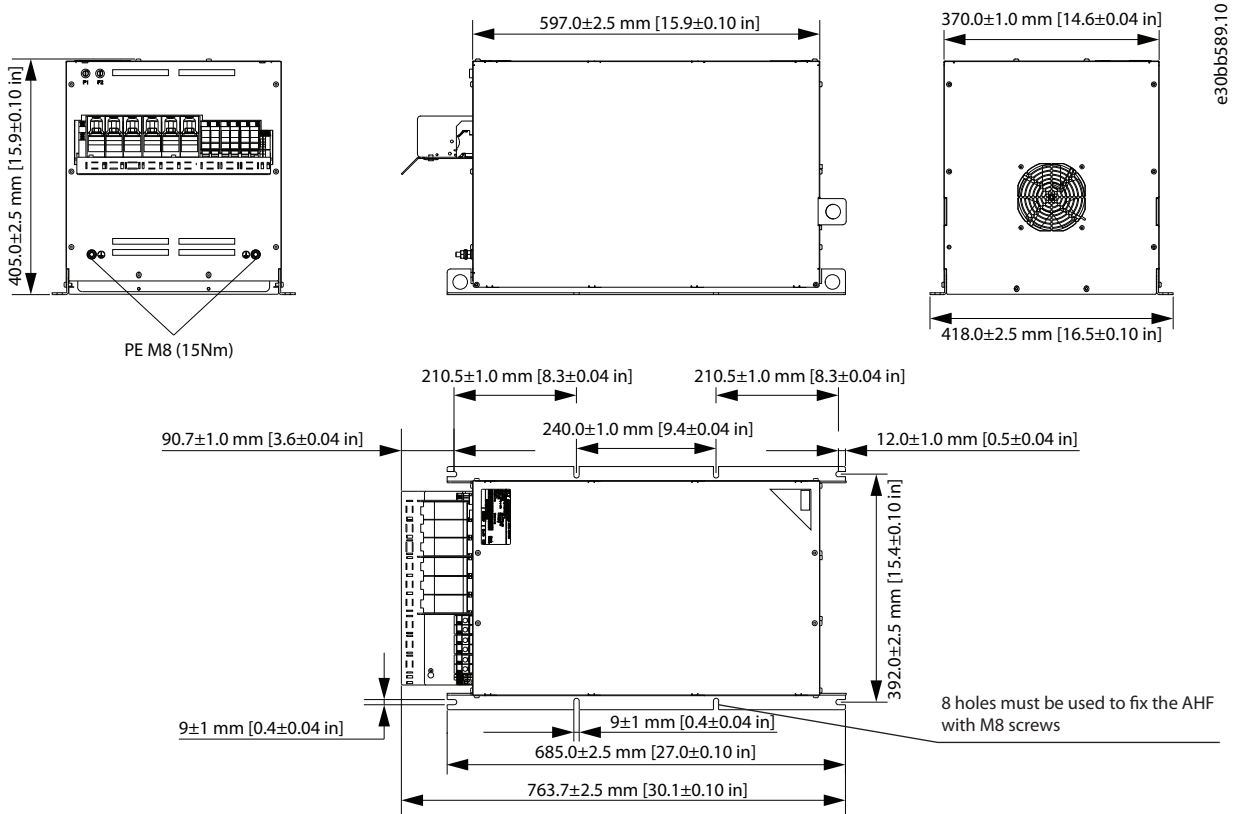
Abbildung 7.22 IP20 X6-V3 Interner Lüfter
