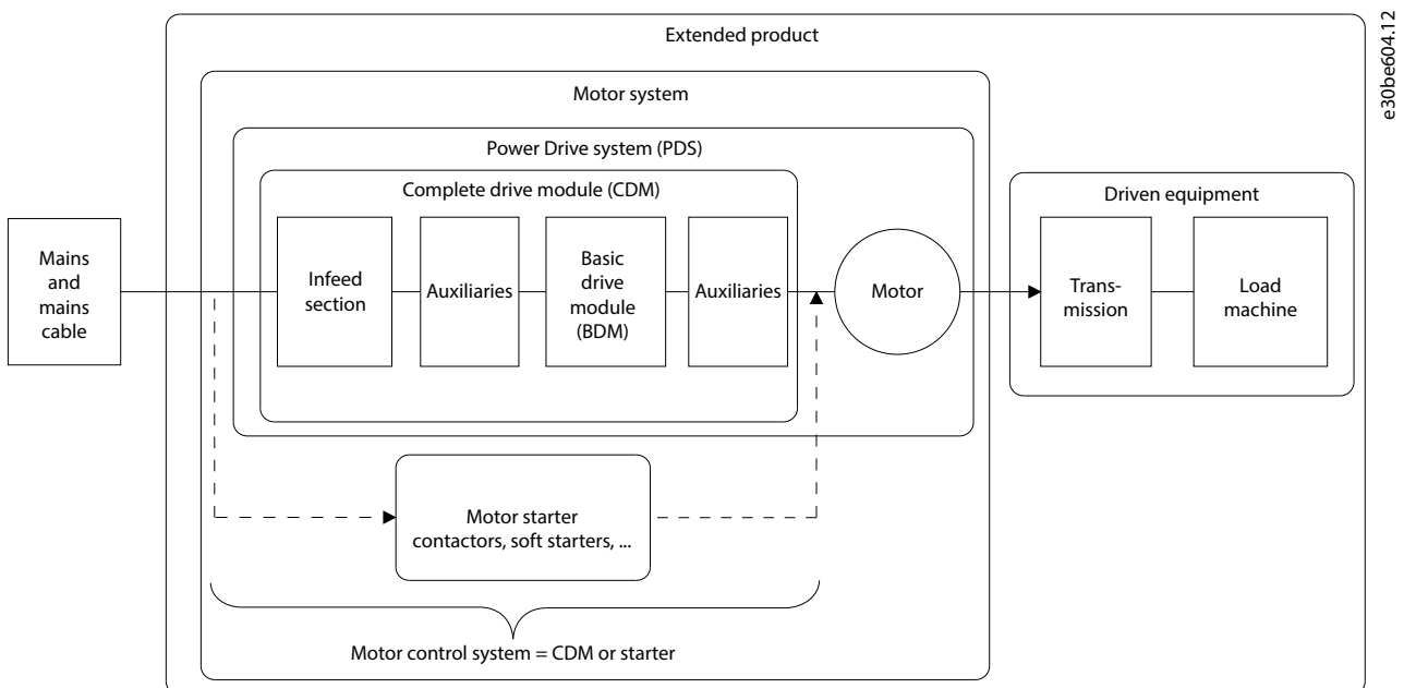
Abbildung 9.1 Antriebssystem und komplettes Antriebsmodul
