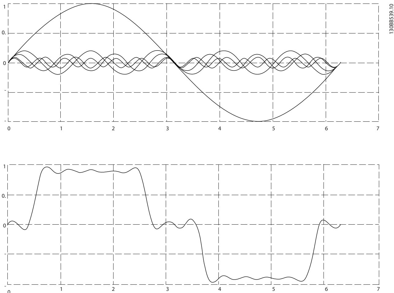
Abbildung 2.3 Sinusförmige Signalkurven
