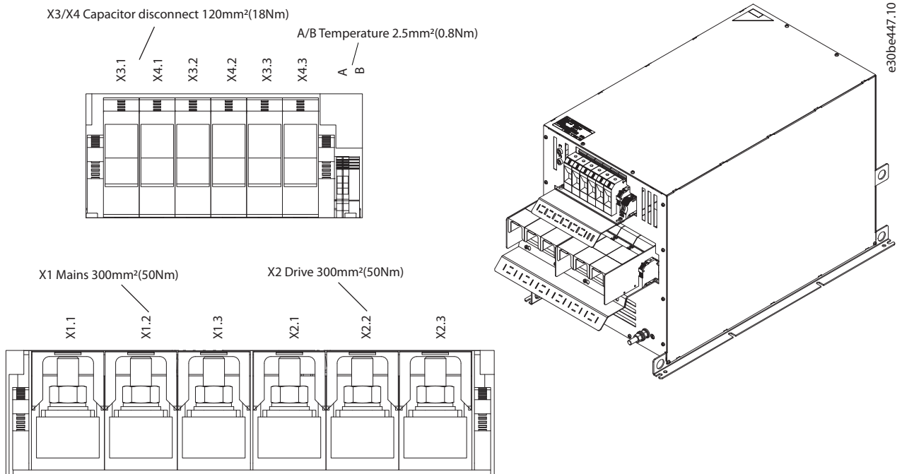
Abbildung 7.31 IP20 X8-V3 Interner Lüfter, Klemmenbezeichnung und 3D-Ansicht
