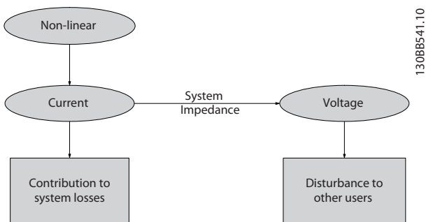
Abbildung 2.5 Die störende Wirkung von Oberschwingungen
