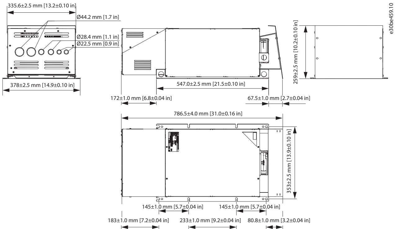
Abbildung 7.38 IP21 X3-V3 interner und externer Lüfter
