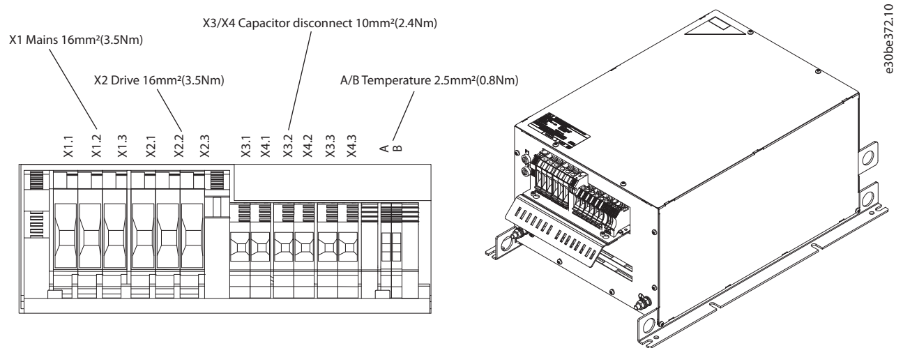
Abbildung 7.11 IP20 X3-V3 Interner Lüfter, Klemmenbezeichnung und 3D-Ansicht
