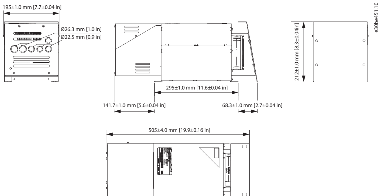
Abbildung 7.34 IP21 X1-V3 interner und externer Lüfter
