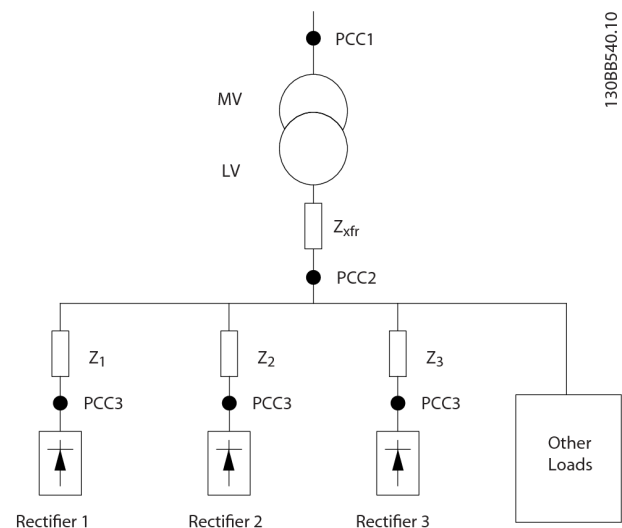
Abbildung 2.4 Kleine Verteilungsanlage
