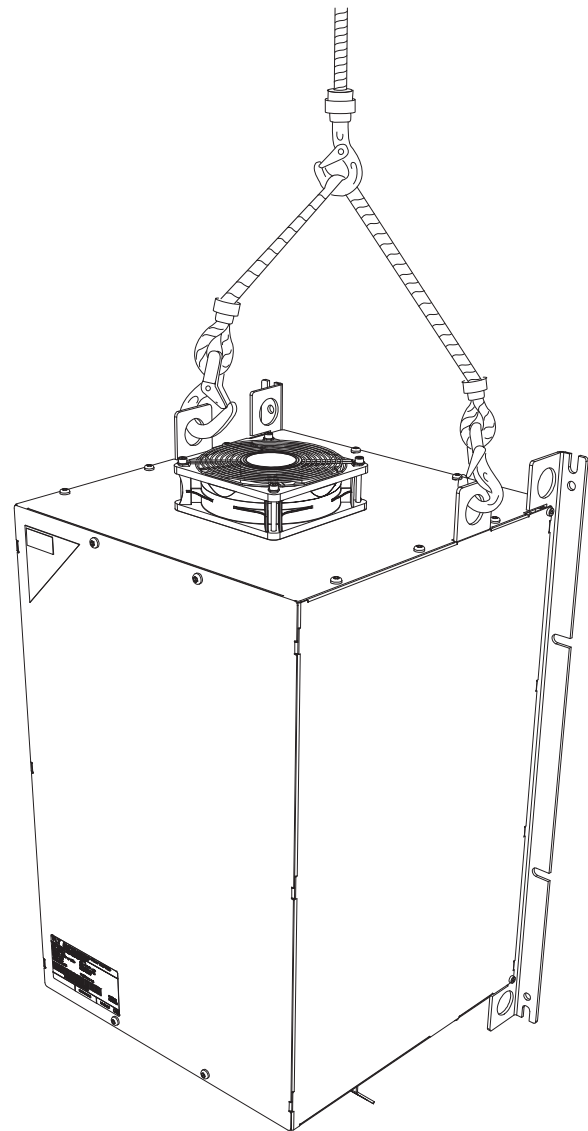
Abbildung 4.2 Empfohlenes Hebeverfahren, Externe Lüfterfilter
