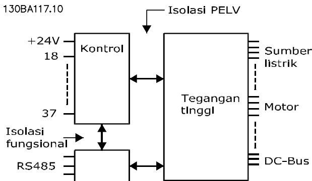
Ilustrasi 10.1 Isolasi PELV
