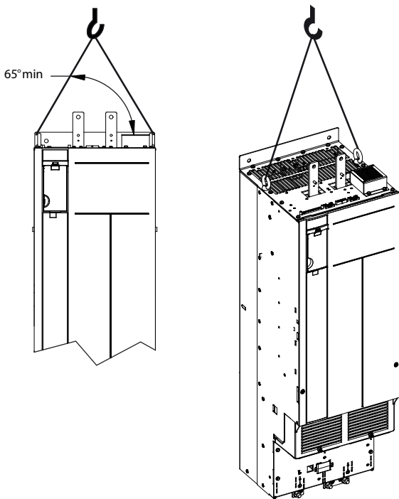
Ilustrasi 4.3 Mengangkat Konverter
