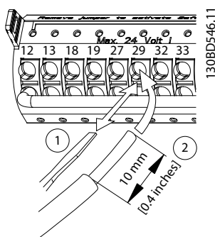
Ilustrasi 5.38 Menghubungkan Kabel Kontrol Fleksibel
