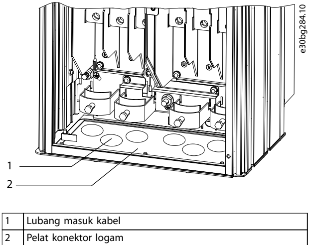
Ilustrasi 4.4 Bukaan Kabel pada Pelat Konektor Logam Lembaran
