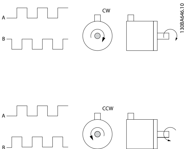
Ilustrasi 8.6 Menentukan Arah Encoder
