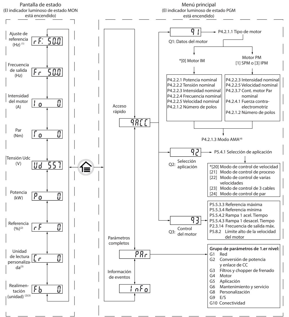
Ilustración 6: Funcionamiento con el panel de control
