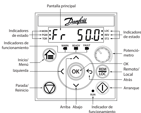
Ilustración 5: Indicadores y teclas de funcionamiento
