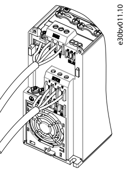
Ilustración 1: Montaje del cable de toma de tierra, de la red eléctrica y de los cables de motor
