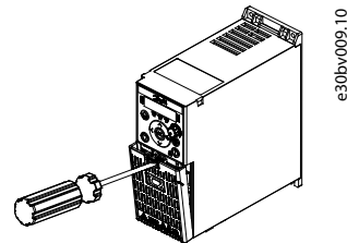
Ilustración 2: Desmontaje de la tapa de terminales
