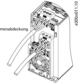
Abbildung 1: Befestigung von Erdungskabel, Netz- und Motorkabeln
