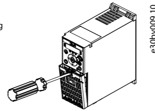
Abbildung 2: Entfernen der Klemmenabdeckung
