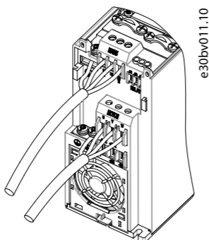
Abbildung 1: Befestigung von Erdungskabel, Netz- und Motorkabeln
