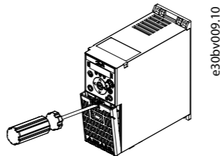
Abbildung 2: Entfernen der Klemmenabdeckung
