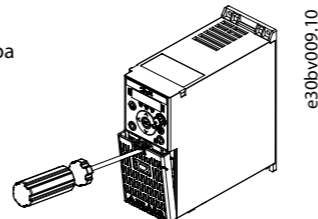
Ilustração 2: Removendo a tampa dos terminais
