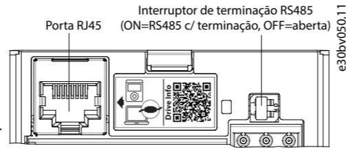
Ilustração 4: Porta RJ45 e chave de terminação RS485
