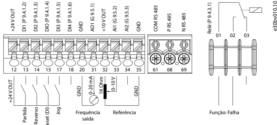
Ilustração 3: Visão Geral dos Terminais de Controle na Configuração PNP com Configuração de Fábrica (Modo de Controle de Velocidade)
