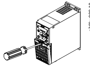
图 2: 拆除端子盖
