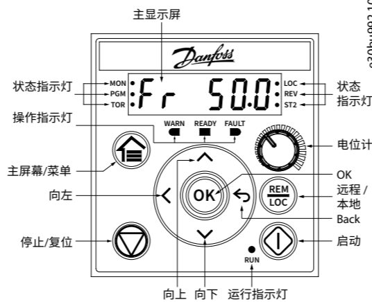
图 5：指示灯和操作按钮
