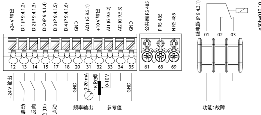
图 3：默认设置为 PNP 配置 (速度控制模式) 的控制端子概述
