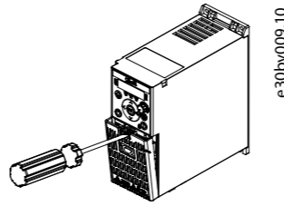
图 2：拆除端子盖
