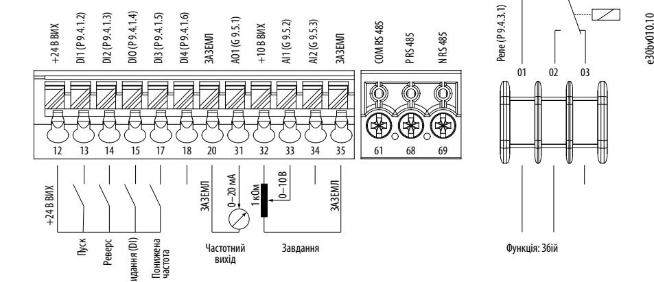
Ілюстрація 3: Огляд клем керування в конфігурації PNP за заводських налаштувань параметрів (Режим регулювання швидкості)
