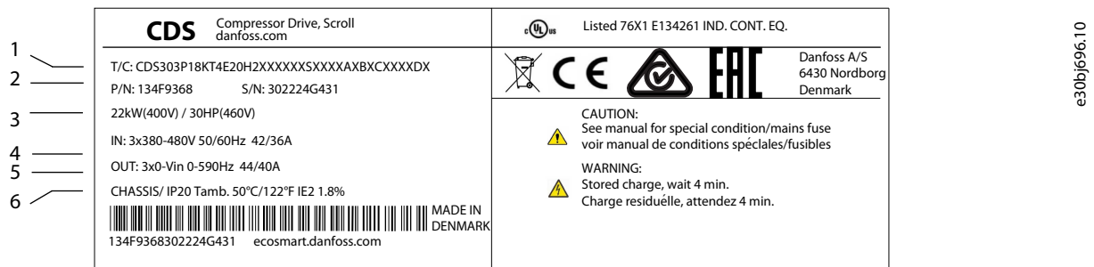
Abbildung 1: Beispiel für den Typencode auf dem Typenschild
