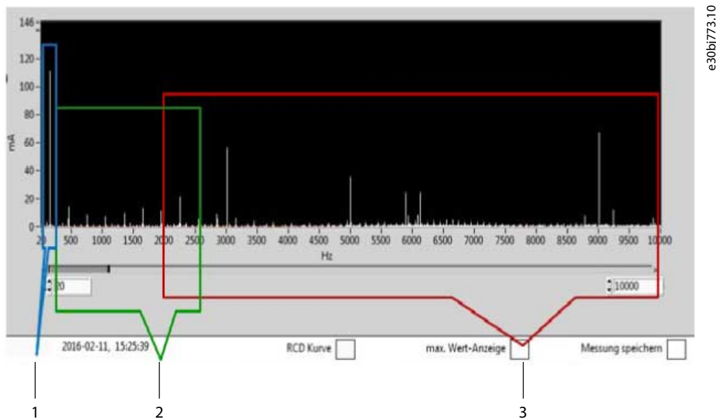
Illustration 29: Exemple de mesure FFT
