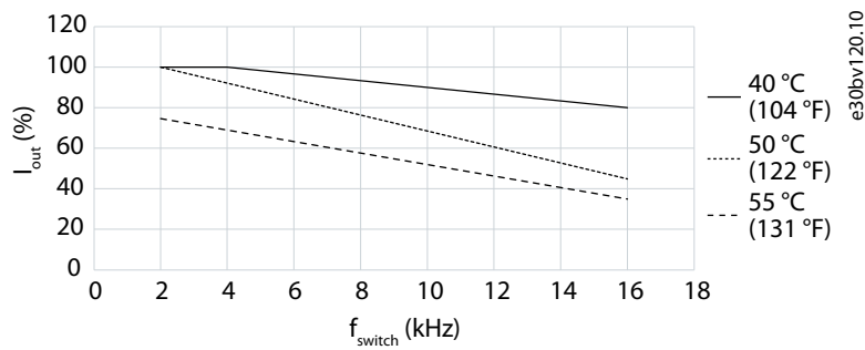
Illustration 16: Déclassement du courant de sortie par rapport à la fréquence de commutation (MA02a 1 x 200-240 V CA)
