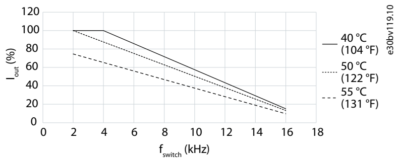
Illustration 15: Déclassement du courant de sortie par rapport à la fréquence de commutation (MA01a 3 x 380-480 V CA)
