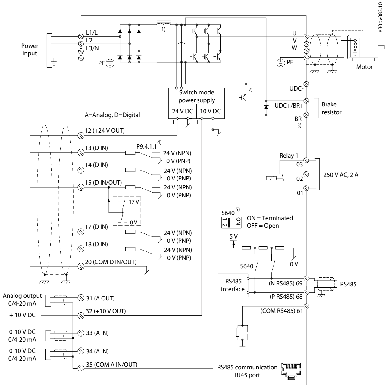
Illustration 28: Schéma de câblage
