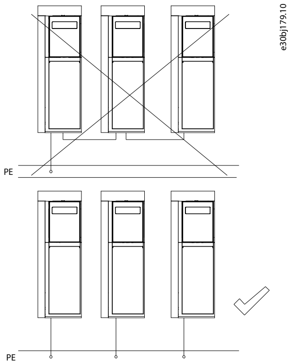
Illustration 32: Principe de mise à la terre
