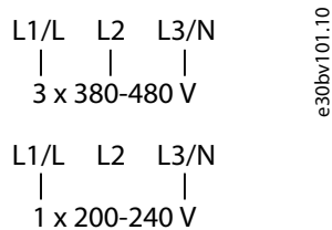
Illustration 39: Raccordements des câbles monophasés et triphasés
