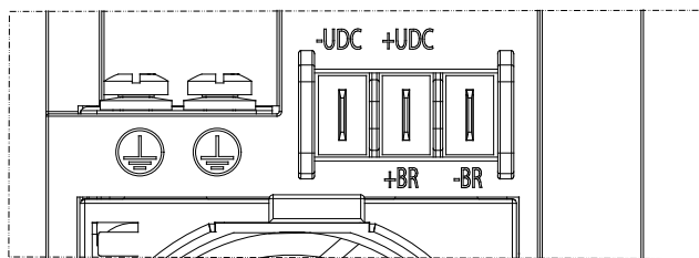
Illustration 45: Fonction de frein de MA02a (3 x 380-480 V)
