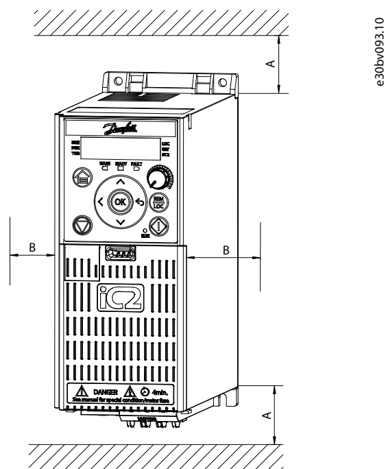
Illustration 26: Dégagement minimum pour le refroidissement
