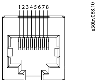
Illustration 7: Définition des broches du RJ45
