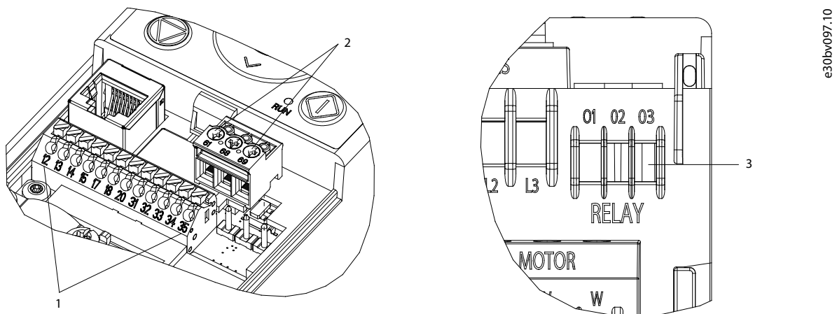
Illustration 40: Numéros et emplacements des bornes de commande
