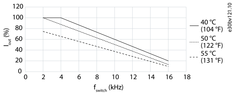
Illustration 17: Déclassement du courant de sortie par rapport à la fréquence de commutation (MA02a 3 x 380-480 V CA)
