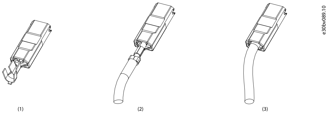
Illustration 43: Câblage du connecteur de répartition de la charge et du frein
