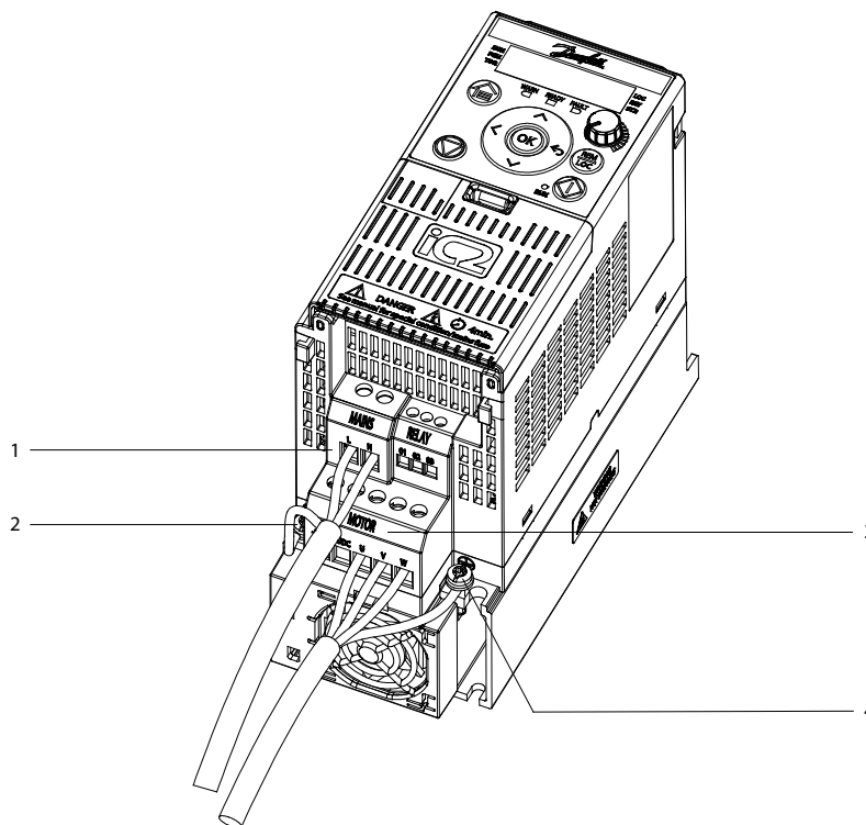
Illustration 37: Raccordement du secteur et du moteur et mise à la terre pour les unités monophasées (exemple : MA02c)
