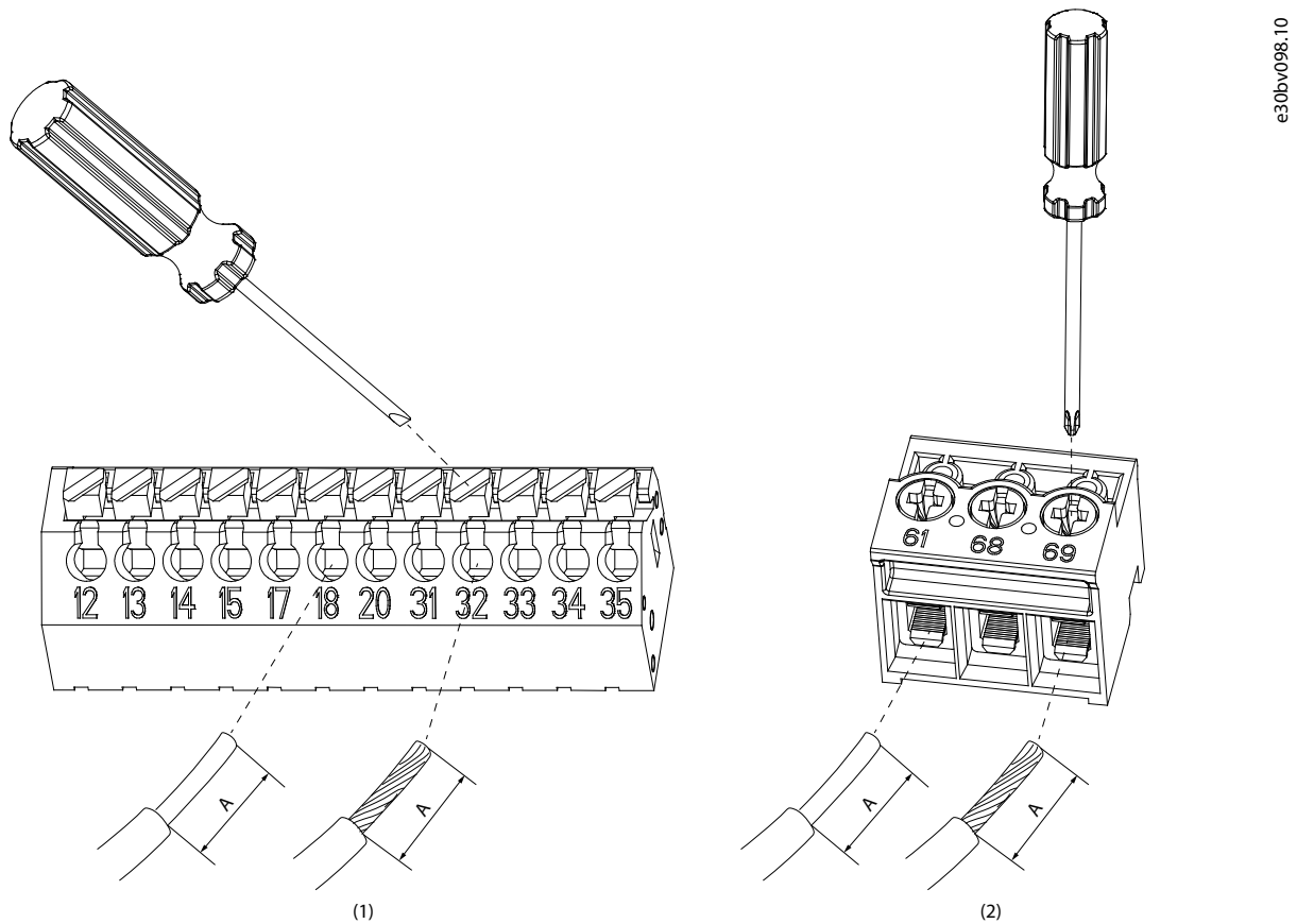
Illustration 41: Insertion des fils dans le connecteur
