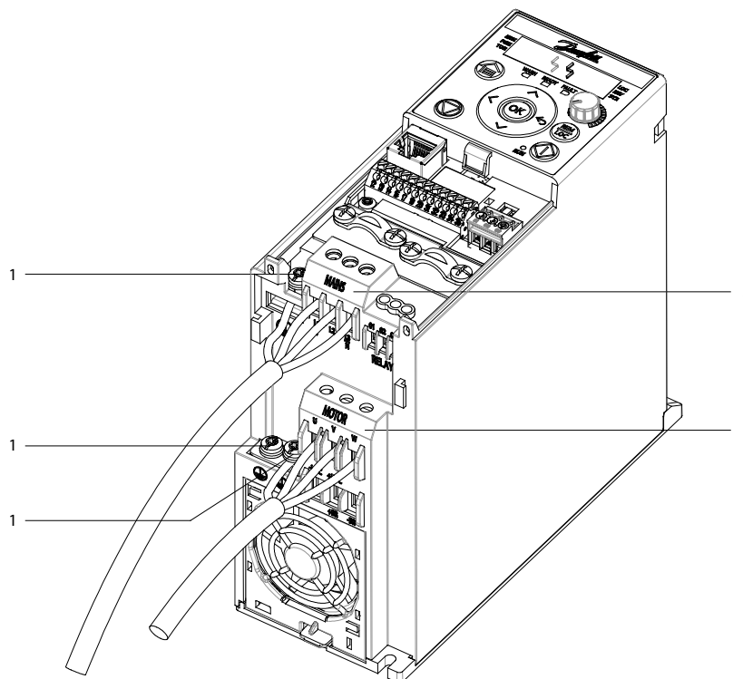
Illustration 38: Mise à la terre et raccordement du secteur et du moteur des unités triphasées (exemple de MA02a)
