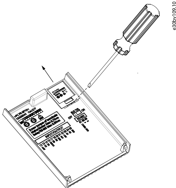
Illustration 10: Retrait de la porte coulissante
