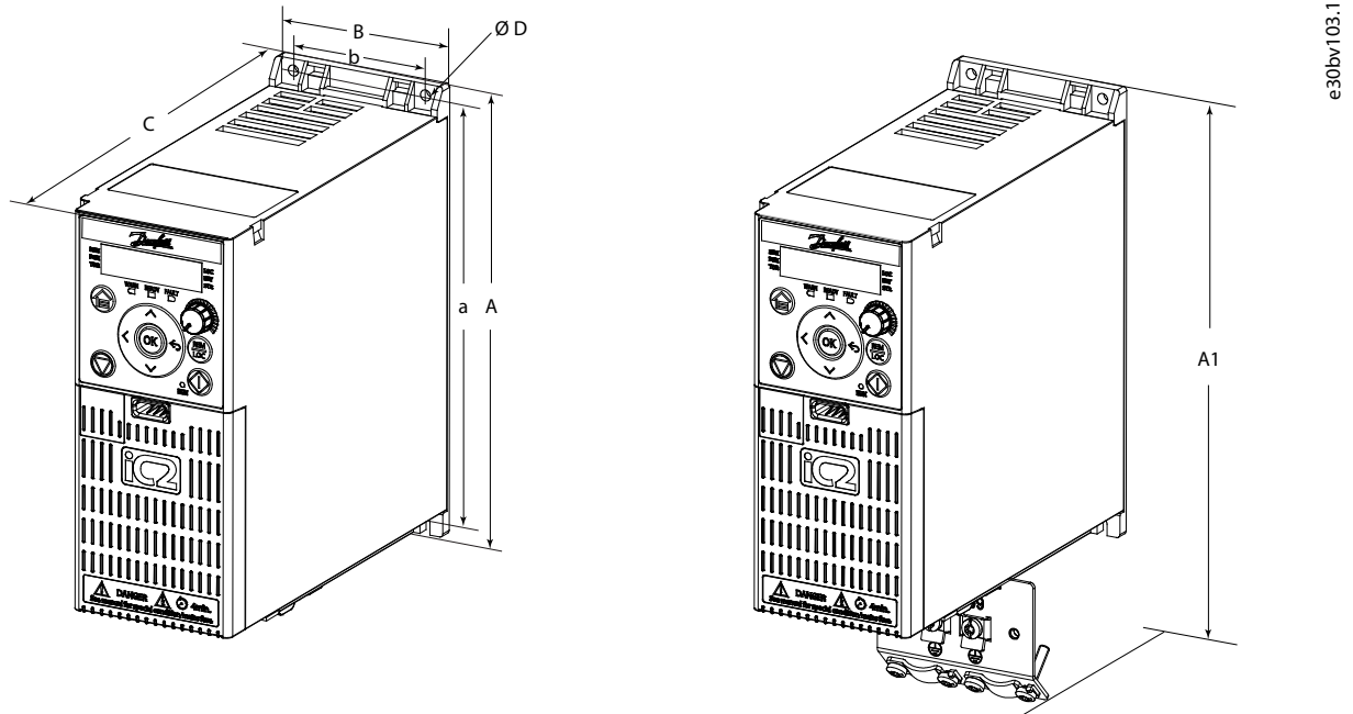
Illustration 18: Tailles et dimensions protection IP20/de type ouvert
