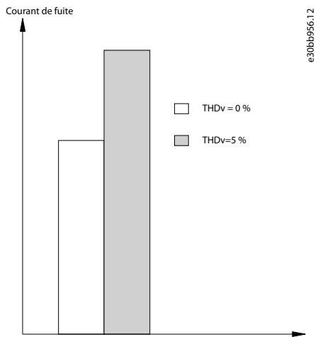
Illustration 35: Influence de la distorsion de la ligne sur le courant de fuite
