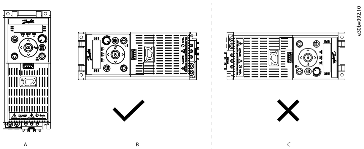
Illustration 24: Sens de montage des variateurs
