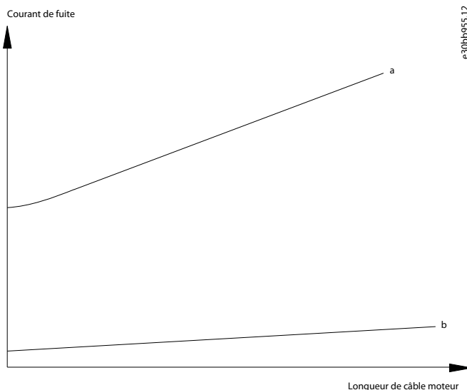
Illustration 34: Influence de la longueur de câble et de la puissance sur le courant de fuite, P_a > P_b
