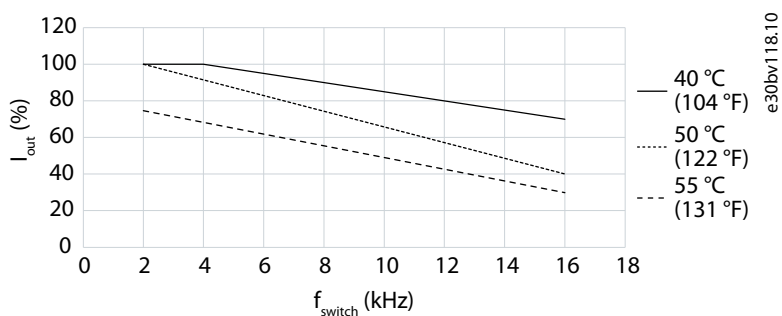
Illustration 14: Déclassement du courant de sortie par rapport à la fréquence de commutation (MA02c 1 x 200-240 V CA)
