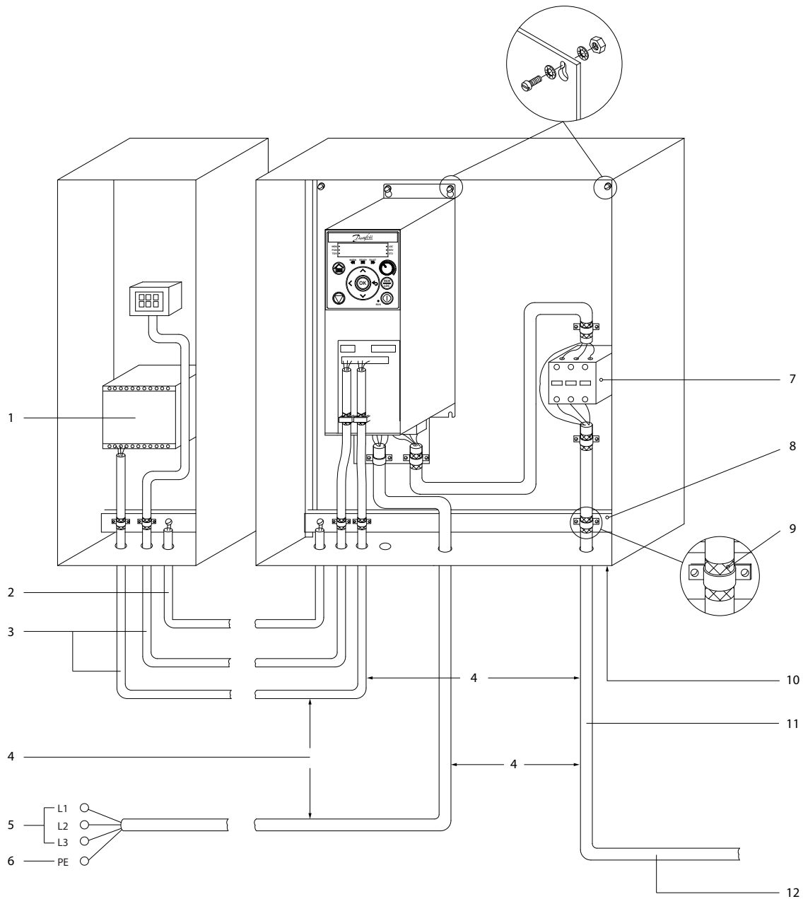
Illustration 30: Exemple d'installation conforme aux exigences CEM
