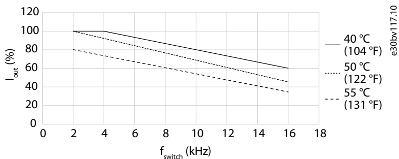
Illustration 13: Déclassement du courant de sortie par rapport à la fréquence de commutation (MA01c 1 x 200-240 V CA)
