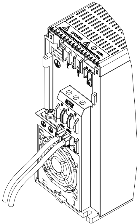
Illustration 44: Connexion à la répartition de la charge et au frein
