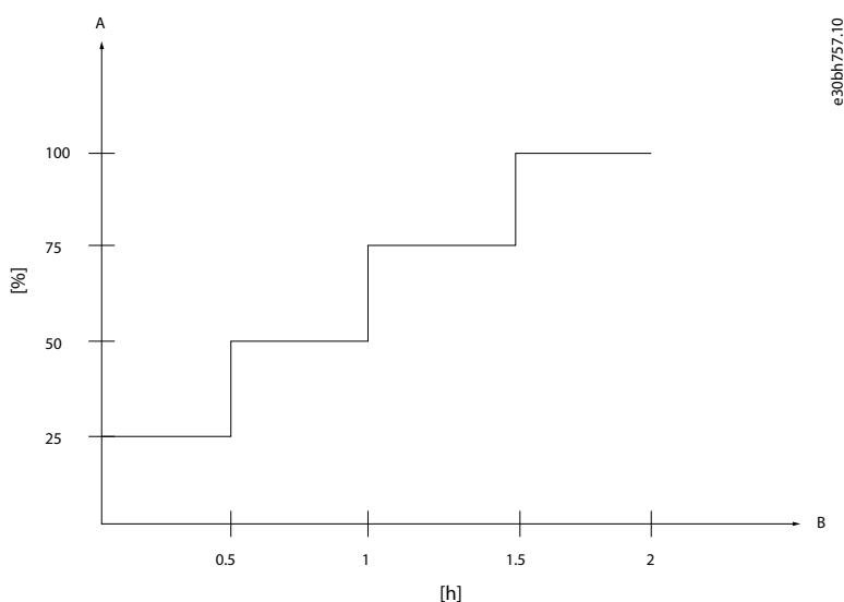
Illustration 23: Procédure de régénération des condensateurs CC
