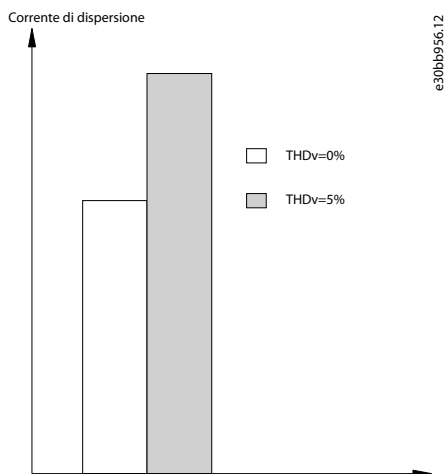
Illustrazione 35: Influsso della distorsione di linea sulla corrente di dispersione
