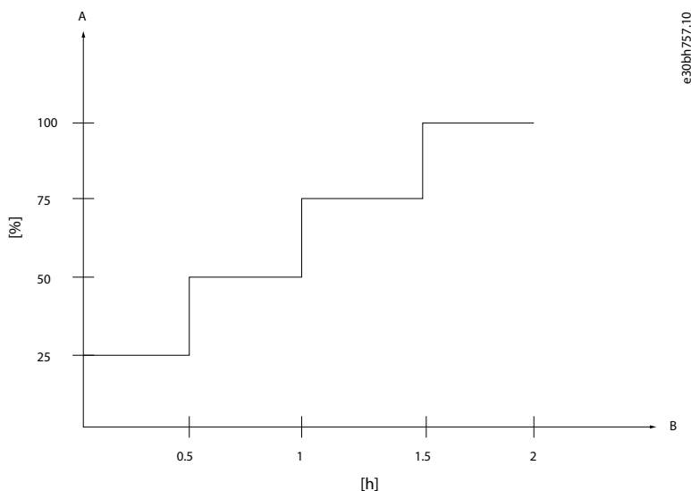
Illustrazione 23: Procedura di rigenerazione per condensatori CC
