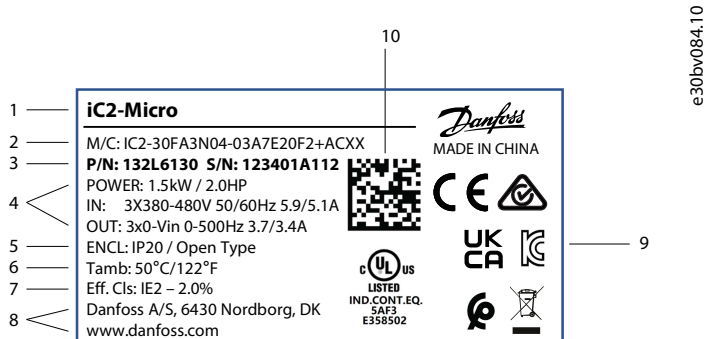
Illustrazione 21: Esempio di etichetta di un prodotto
