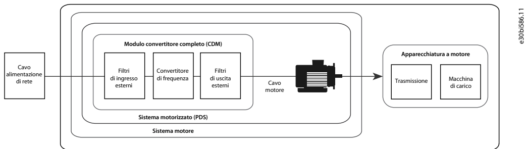
Illustrazione 3: Progettazione del sistema convertitore
