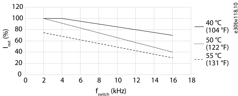
Illustrazione 14: Declassamento della corrente di uscita rispetto alla frequenza di commutazione (MA02c 1x200-240 V CA)
