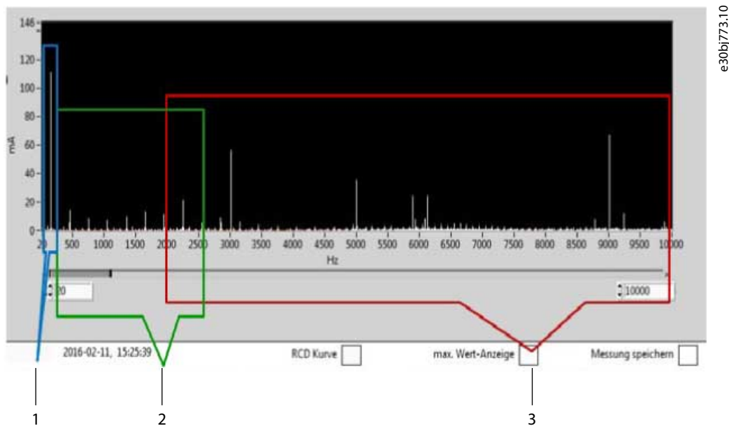
Illustrazione 29: Esempio di misurazione FFT
