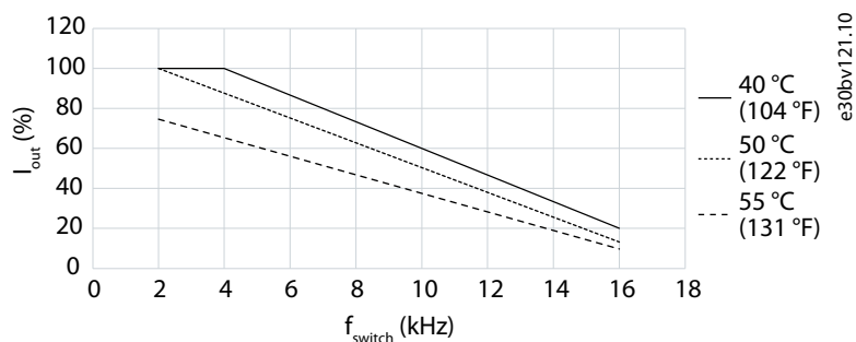
Illustrazione 17: Declassamento della corrente di uscita rispetto alla frequenza di commutazione (MA02a 3x380-480 V CA)
