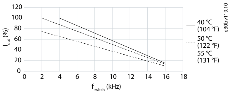
Illustrazione 15: Declassamento della corrente di uscita rispetto alla frequenza di commutazione (MA01a 3x380-480 V CA)
