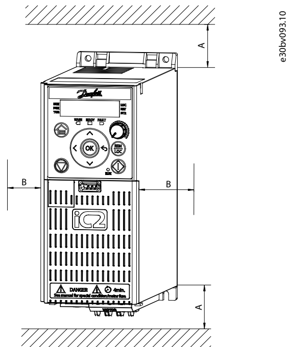
Illustrazione 26: Spazio minimo per il raffreddamento
