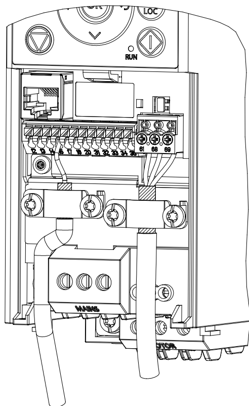
Illustrazione 42: Collegamento corretto dello schermo del cavo
