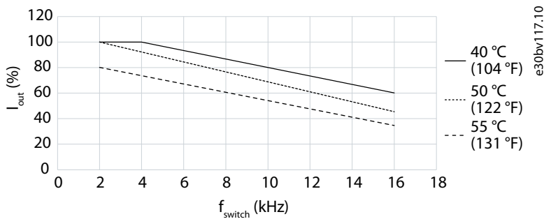
Illustrazione 13: Declassamento della corrente di uscita rispetto alla frequenza di commutazione (MA01c 1x200-240 V CA)
