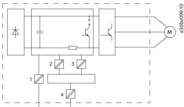
Illustrazione 33: Isolamento galvanico
