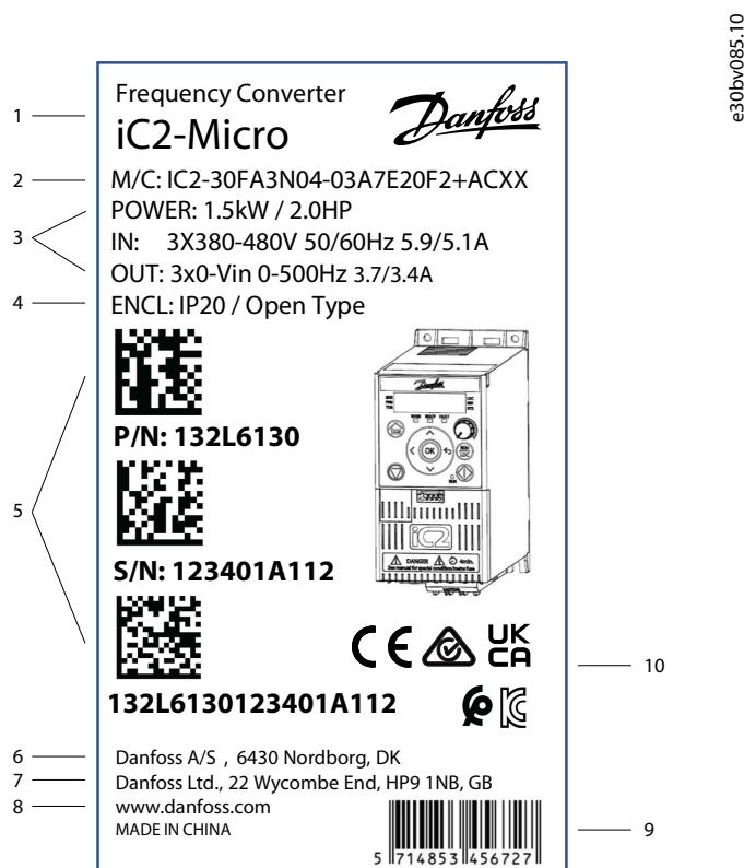
Illustrazione 22: Esempio di etichetta di imballo
