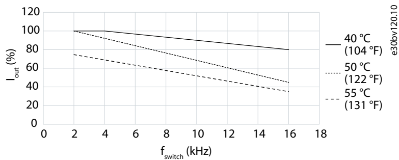
Illustrazione 16: Declassamento della corrente di uscita rispetto alla frequenza di commutazione (MA02a 1x200-240 V CA)
