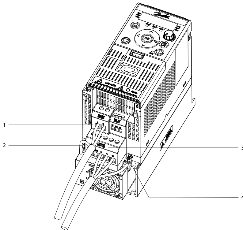
Illustrazione 37: Collegamento di rete, motore e messa a terra per unità monofase (prendendo come esempio MA02c)
