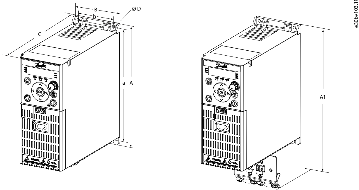
Illustrazione 18: Taglie e dimensioni del contenitore IP20/tipo aperto
