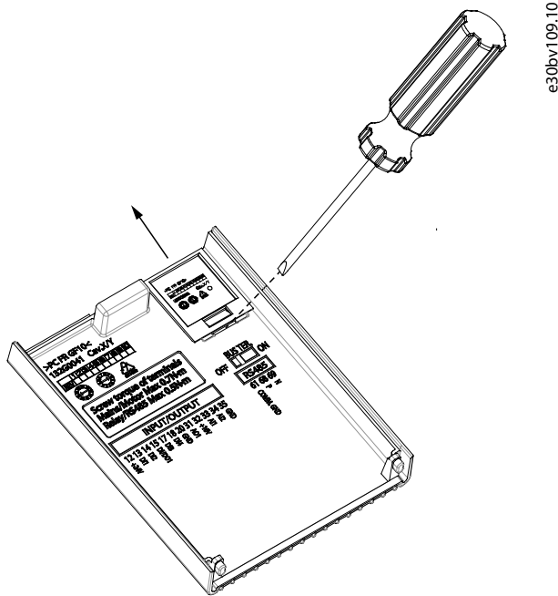
Illustrazione 10: Rimozione dello sportello scorrevole
