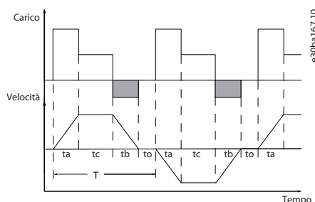
Illustrazione 12: Ciclo di frenatura tipico
