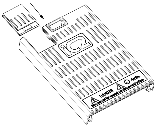
Illustrazione 11: Installazione dello sportello scorrevole
