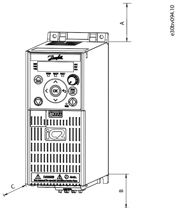
Illustrazione 27: Spazio libero consigliato per l'accesso per la manutenzione
