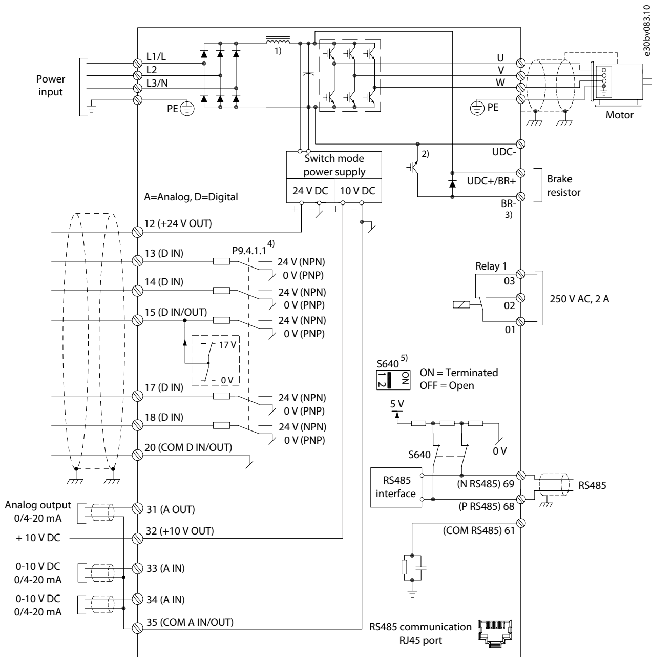
Illustrazione 28: Schema di cablaggio
