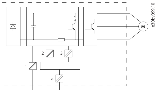
Ilustração 36: Isolação Galvânica
