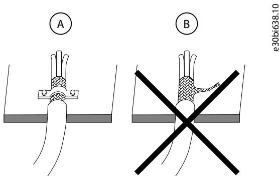
Ilustração 34: Instalação da blindagem do cabo
