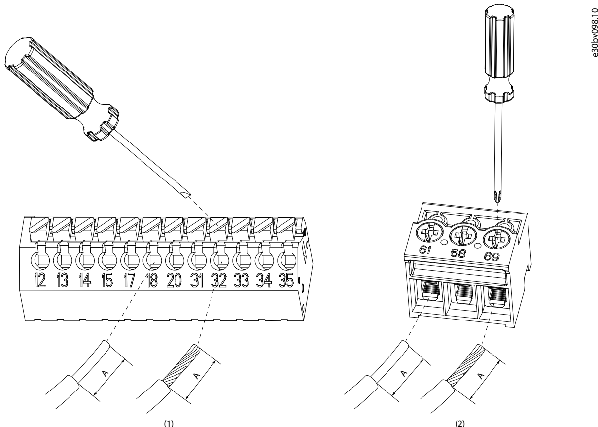
Ilustración 44: Inserción de cables en el conector
