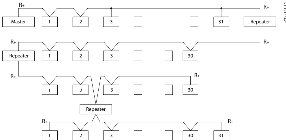
Abbildung 49: RS485-Busschnittstelle
