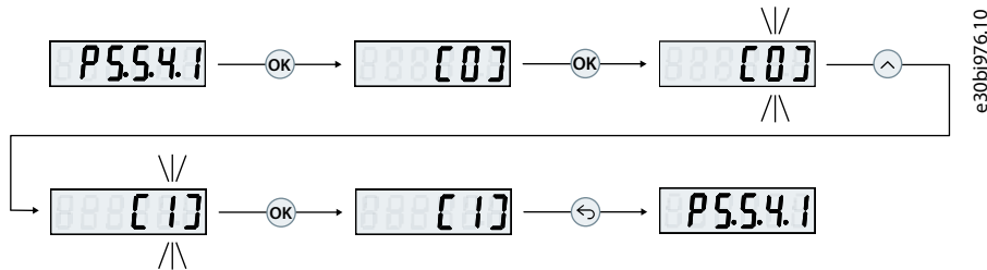
Abbildung 7: Ändern der Auswahl bei einem Parameter
