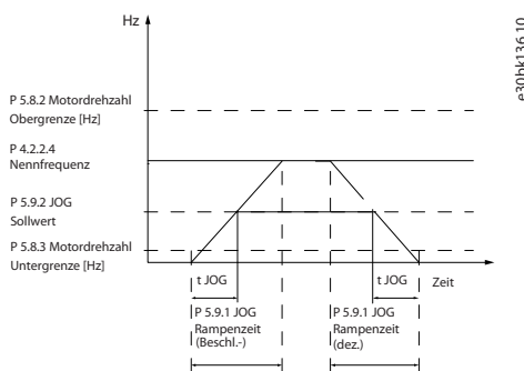
Abbildung 75: Rampenzeit JOG
