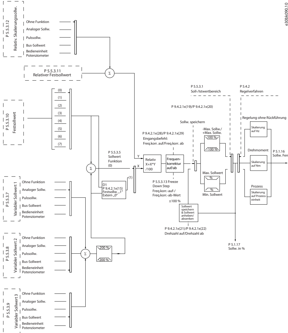
Abbildung 41: Fernsollwert
