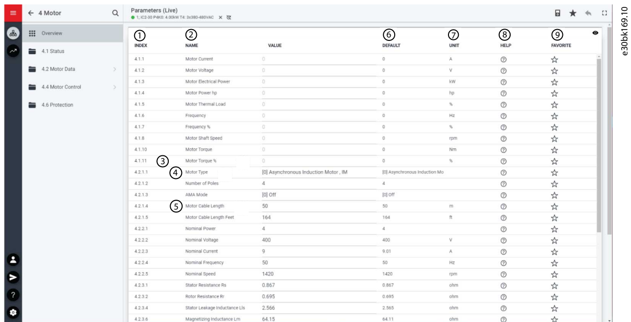
Abbildung 25: Parameterübersicht
