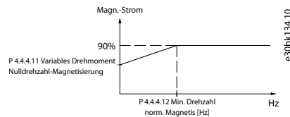
Abbildung 69: Motormagnetisierung
