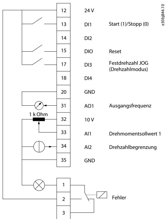
Abbildung 40: Standardanschlüsse
