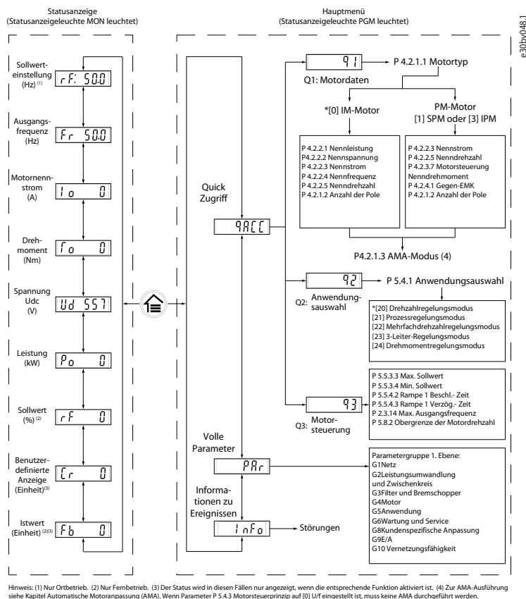
Abbildung 2: Betrieb mit der Bedieneinheit
