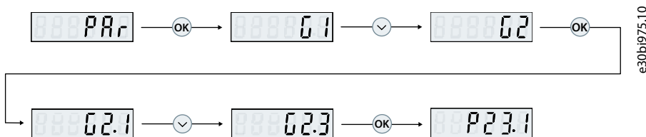
Abbildung 6: Parameternavigation
