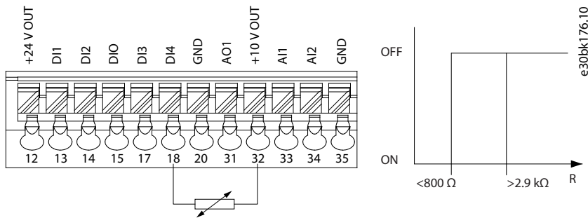
Abbildung 71: PTC-Thermistorverbindung – Digitaleingang
