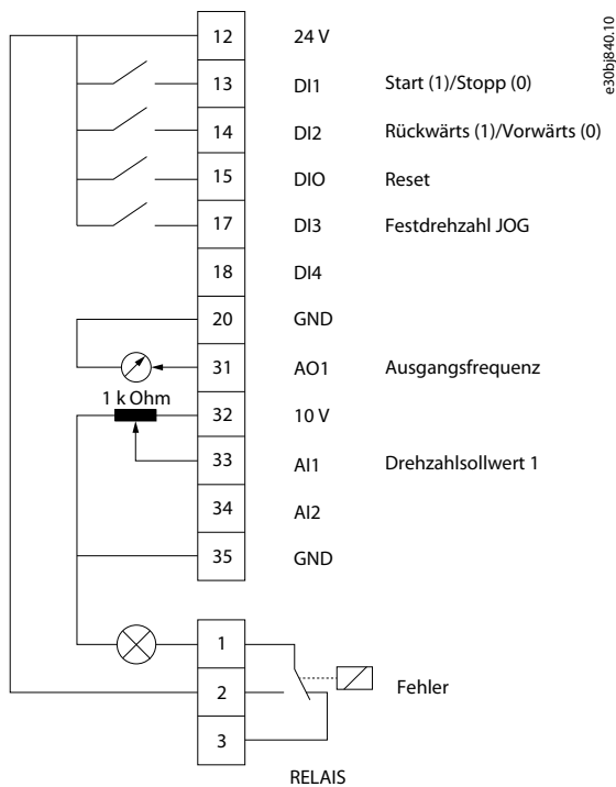
Abbildung 35: Standardanschlüsse
