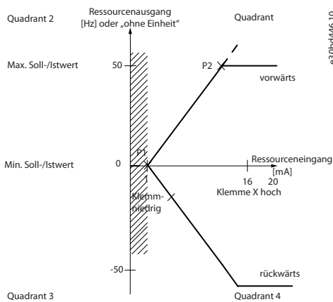
Abbildung 46: Größe der Totzone
