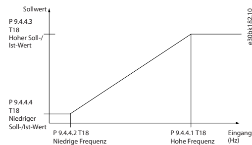
Abbildung 79: Pulseingang
