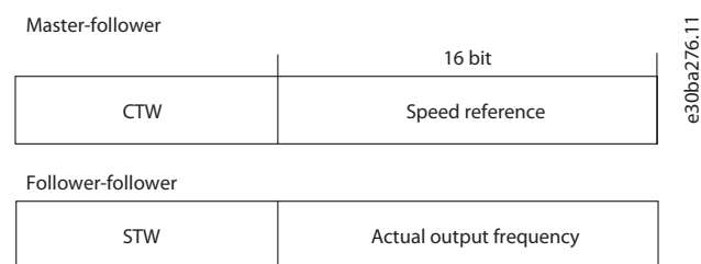
Abbildung 65: Aktuelle Ausgangsfrequenz (HIW)
