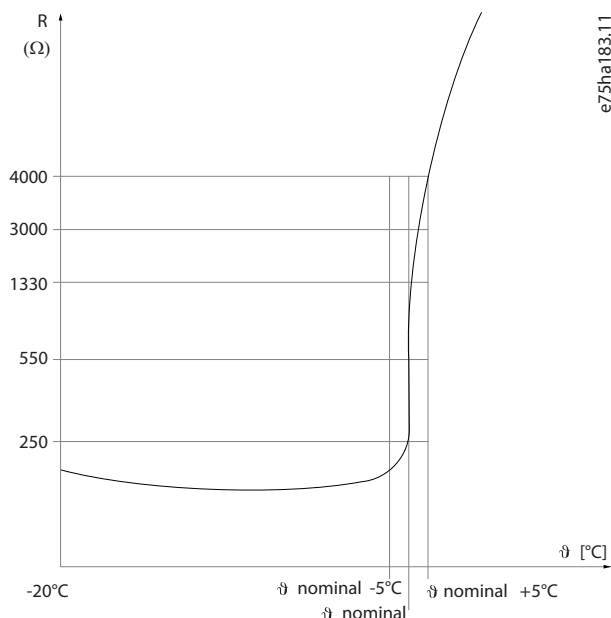
Abbildung 70: PTC-Profil
