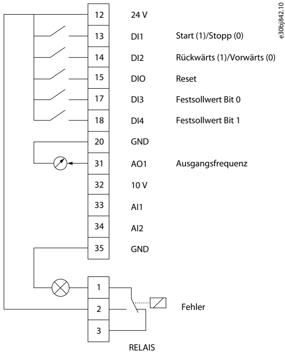
Abbildung 37: Standardanschlüsse
