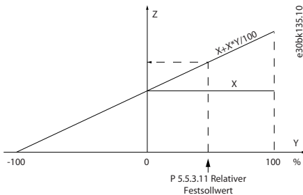
Abbildung 74: Aktueller Sollwert
