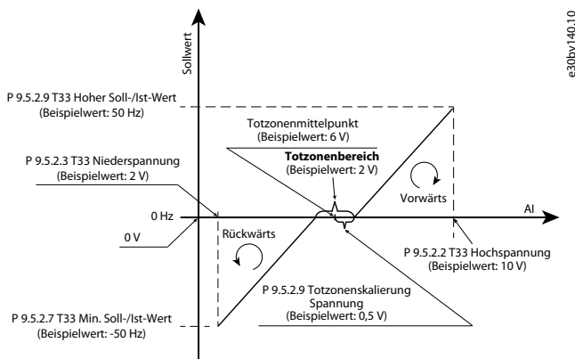
Abbildung 81: Beispiel Totzonenfunktion
