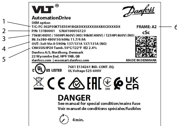
Kuva 1: Esimerkki tyyppikilvestä
