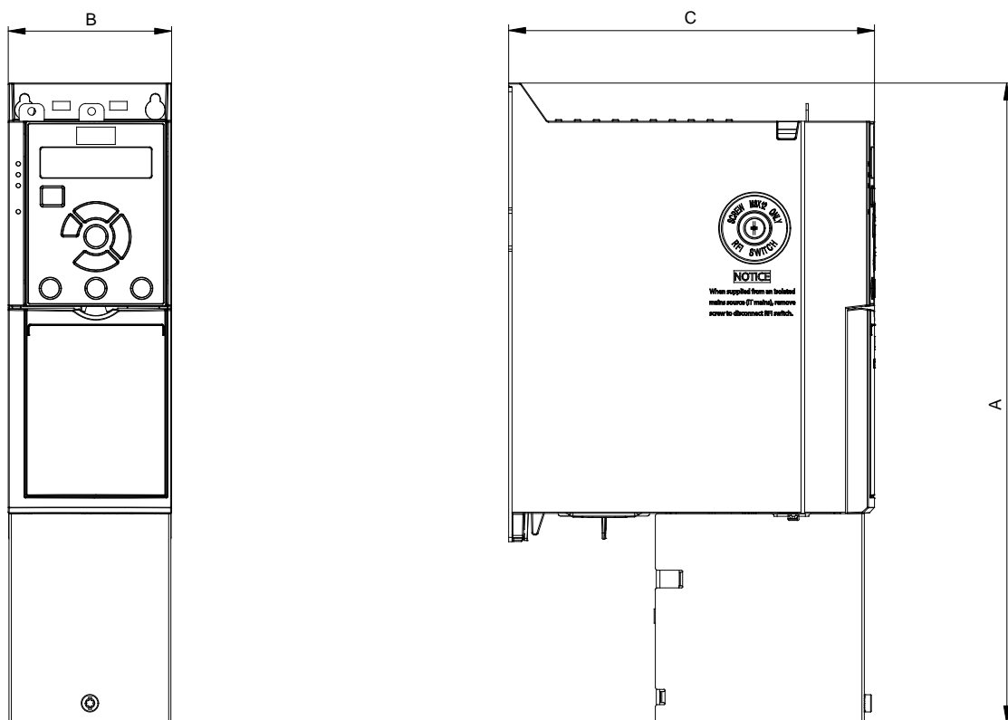
Ilustración 17: Estándar con tapa inferior de entrada de cable (sin tapa superior)
