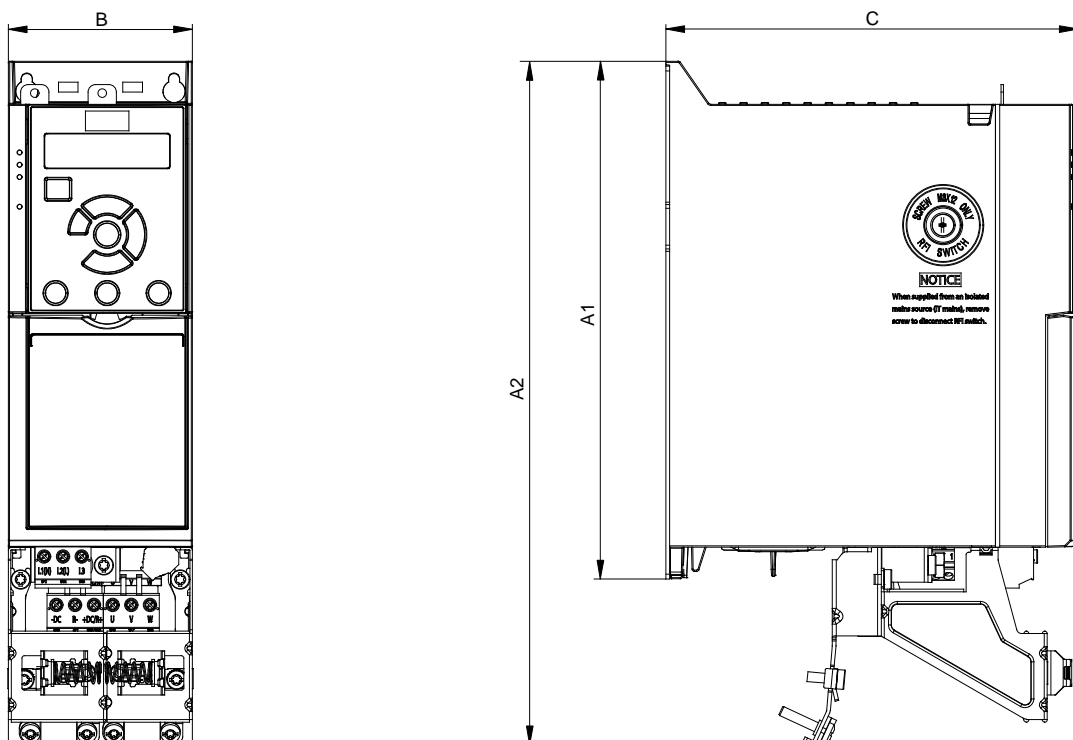
Ilustración 16: Estándar con placa de desacoplamiento
