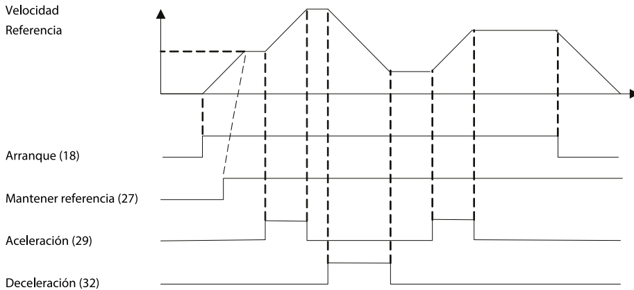
Ilustración 36: Aceleración/deceleración
