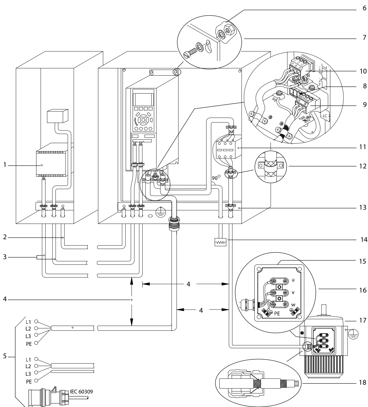
Ilustración 28: Conexión eléctrica típica
