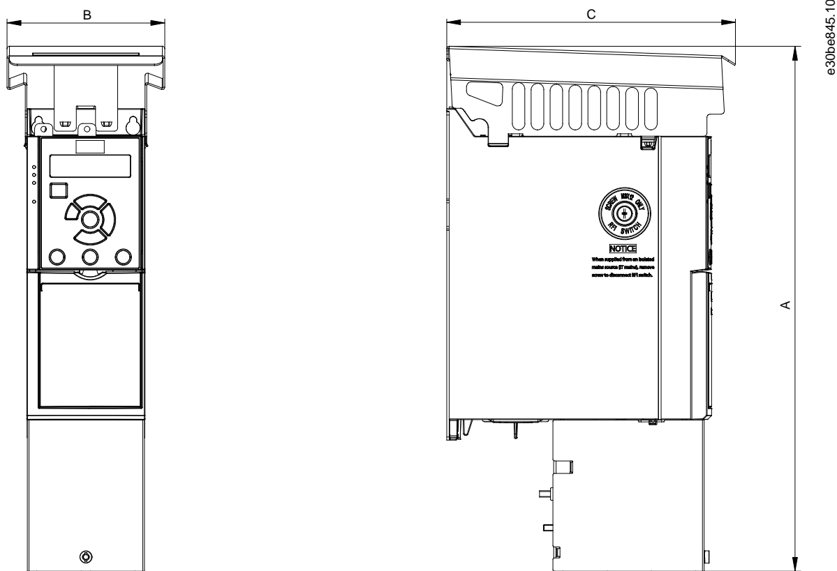
Ilustración 18: Estándar con kit IP21/UL/Tipo 1
