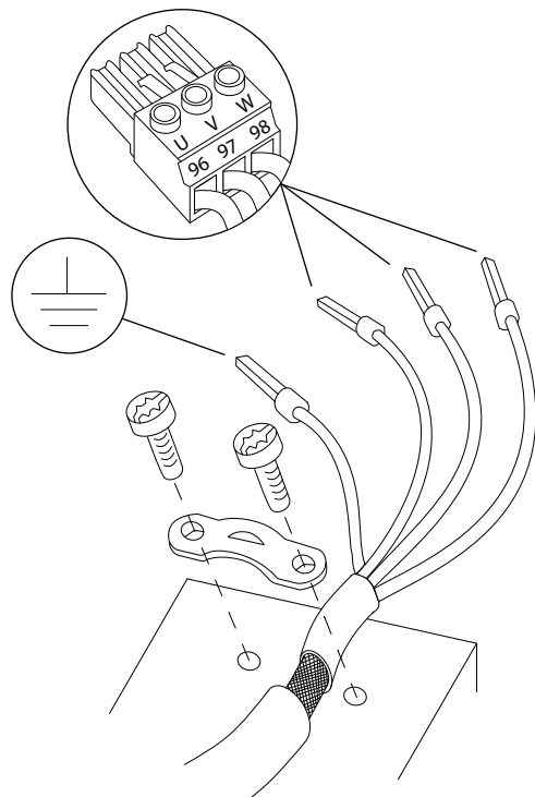
Illustrazione 30: Collegamento del motore
