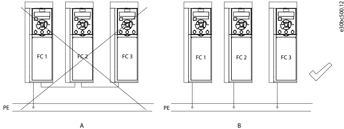
Illustrazione 29: Equalizzazione potenziale di messa a terra
