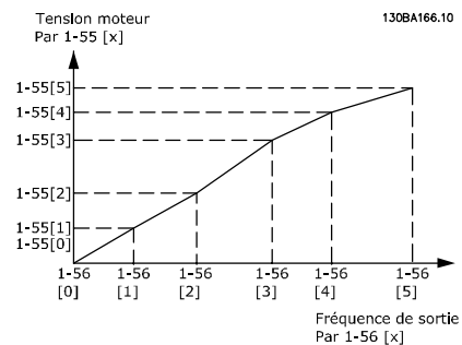
Illustration 4.1 Caractéristique U/f
