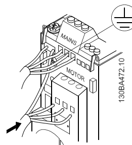
Ilustração 6.7 Montagem do cabo do ponto de aterramento e dos cabos do motor.
