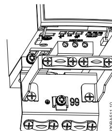
Ilustração 6.8 Conversor de frequência com placa de desacoplamento
