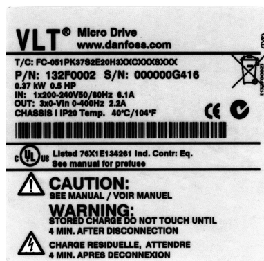
Ilustração 5.1 Este exemplo exibe um adesivo de identificação.
