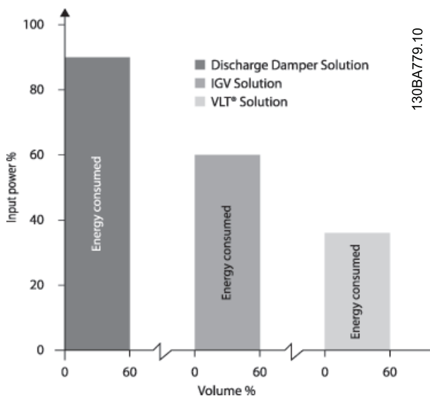
Ilustração 2.5 Economia de Energia
