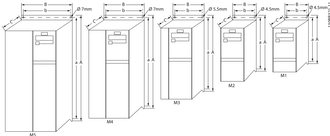
Ilustração 6.3 Dimensões Mecânicas
