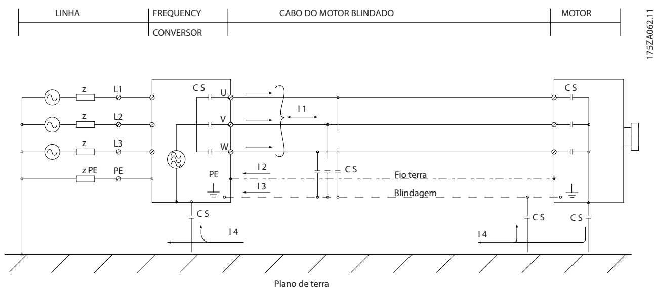
Ilustração 3.3 Situação que Gera Correntes de Fuga
