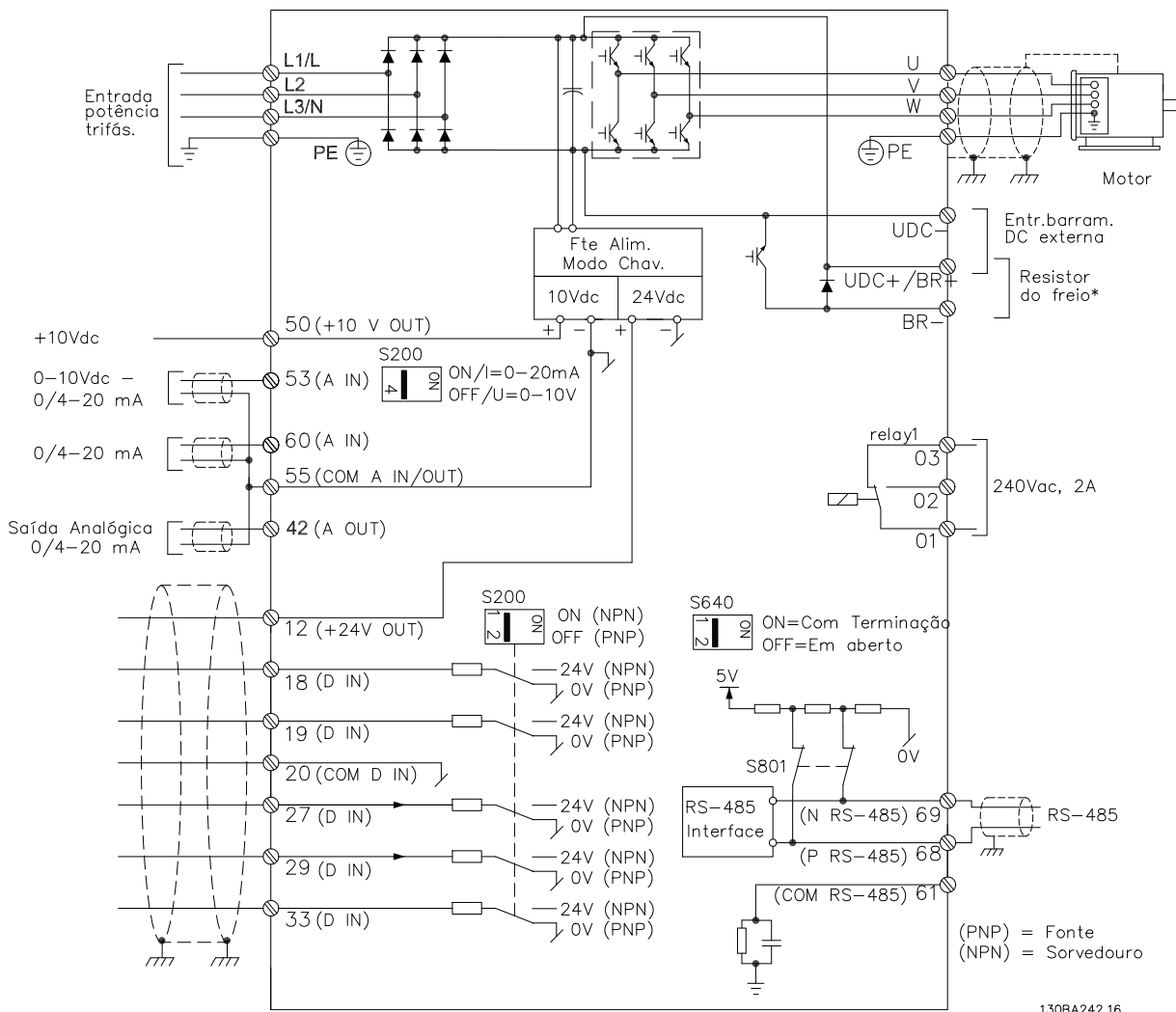
Ilustração 6.10 Diagrama que Mostra todos os Terminais Elétricos
