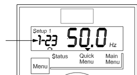
Ilustração 7.4 Indicando Número do Parâmetro Selecionado.
