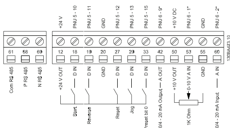
Ilustração 6.12 Visão geral dos terminais de controle na configuração PNP e configuração de fábrica.
