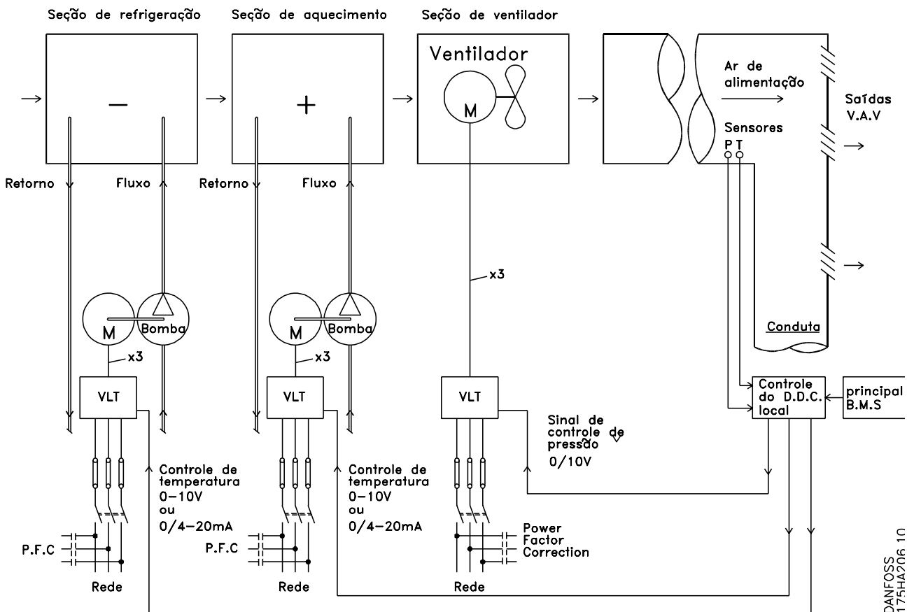
Ilustração 2.6 Sistema de Ventiladores Controlado por Conversores de Frequência
