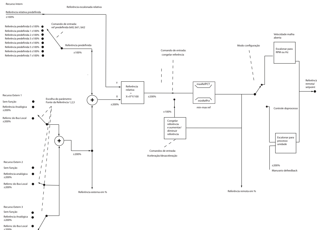
Ilustração 3.2 Diagrama em Bloco Mostrando Referência Remota
