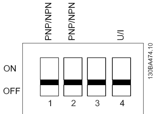
Ilustração 6.14 Chaves S200 1-4.
