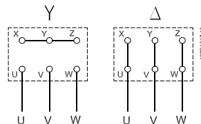
Ilustração 6.6 Conexões delta e em estrela.
