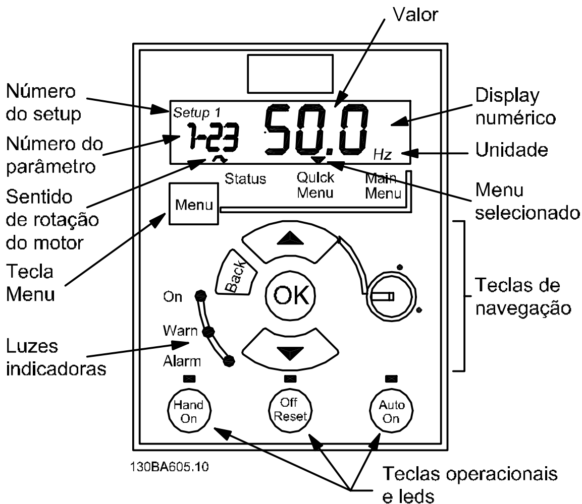
Ilustração 4.1 Descrição dos Botões e do Display do LCP
