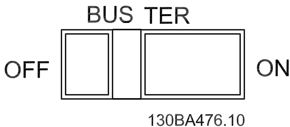
Ilustração 6.13 S640 Terminação do barramento
