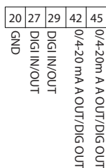
Illustration 4.11 Styreklemmer
