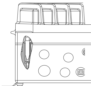
Afbeelding 2.18 Aardverbinding tussen de installatiekast en het elektronische gedeelte
