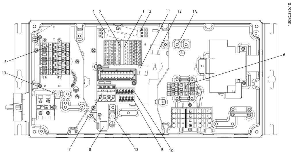
Afbeelding 2.13 Positie van de klemmen (grote eenheden)
