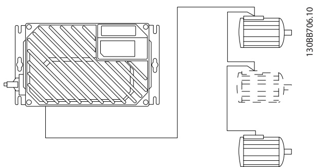
Afbeelding 2.15 Parallele aansluiting van motoren
