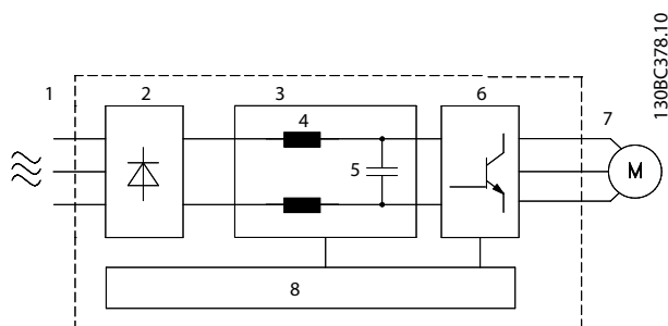
Afbeelding 1.1 Blokschema frequentieomvormer
