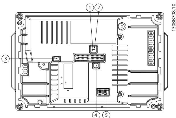
Afbeelding 2.25 Positie van DIP-switches
