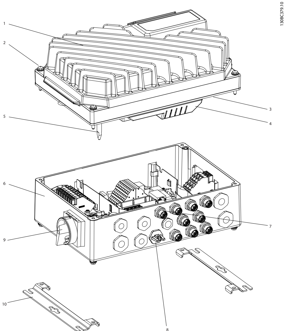
Afbeelding 2.1 Opengewerkte tekening kleine eenheden
