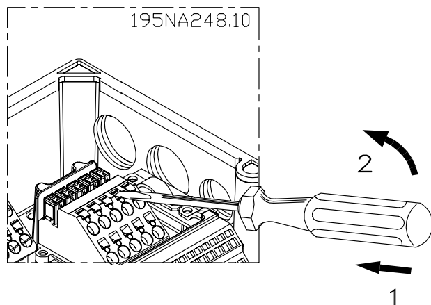
Afbeelding 2.14 De klemmen openen
