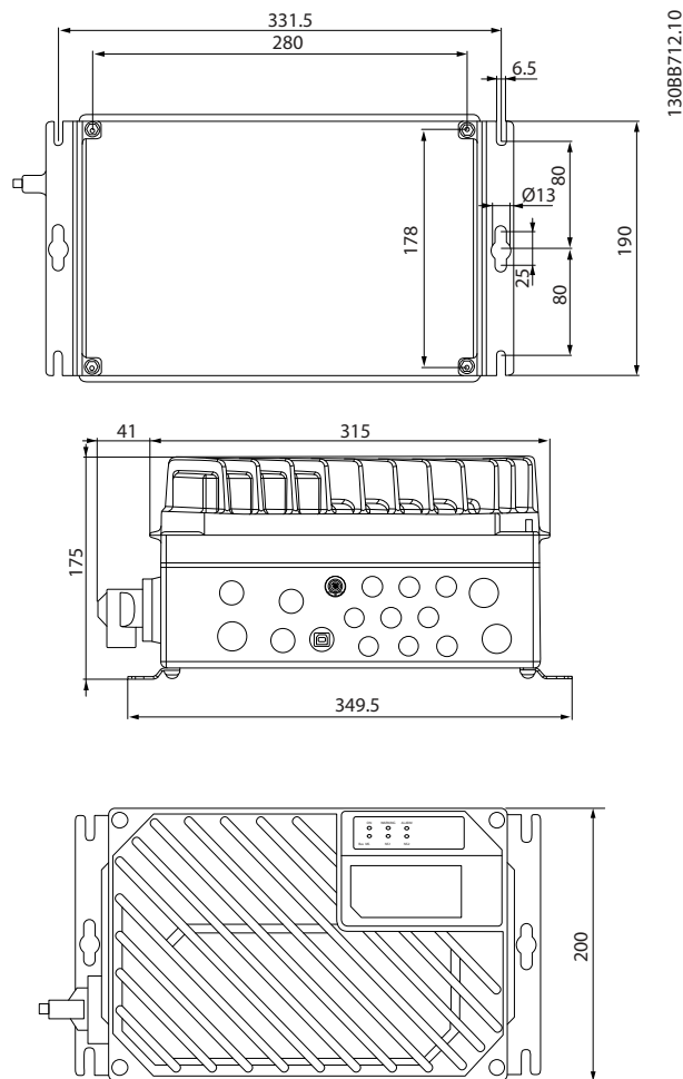
Afbeelding 2.3 Kabeldoorvoeren en gatdiameter (kleine eenheden)
