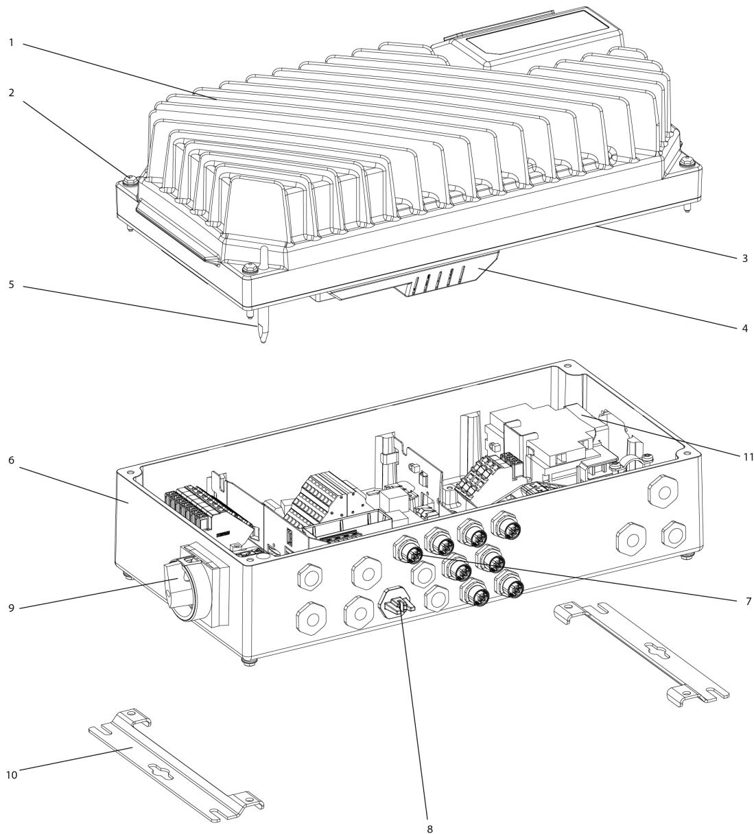
Afbeelding 2.2 Opengewerkte tekening grote eenheid
