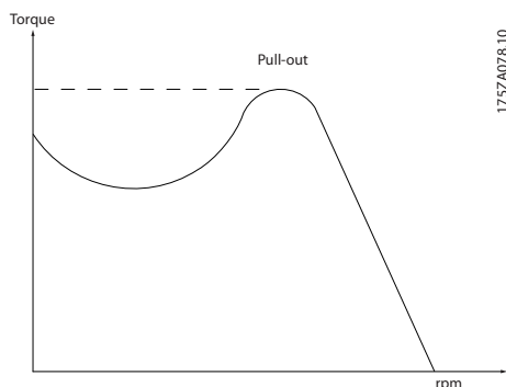
图 1.2 最小启动转矩
