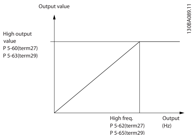
图 4.14 脉冲输出的配置
