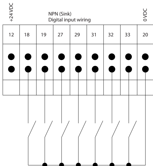
图 1.5 NPN (漏型)
