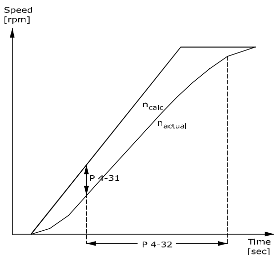
图 4.10 电机反馈速度错误
