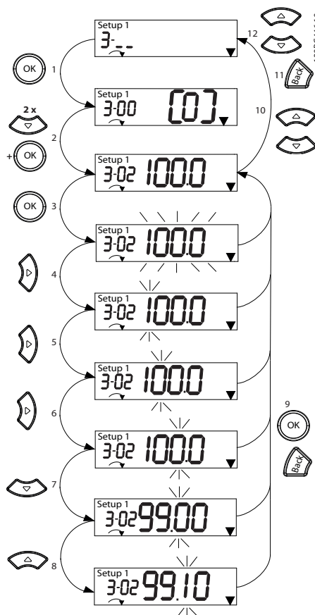
图 3.6 使用主菜单 — 连续参数
