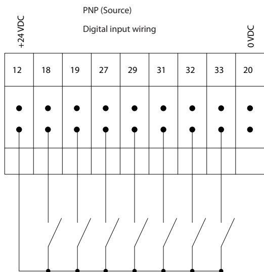
图 1.4 PNP (源型)
