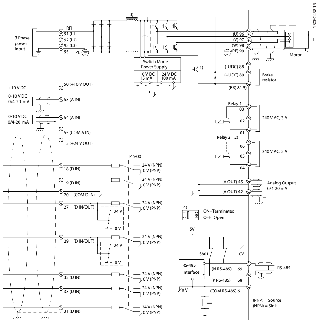
图 1.3 基本接线示意图
