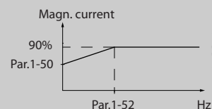
图 4.2 电动机磁化
