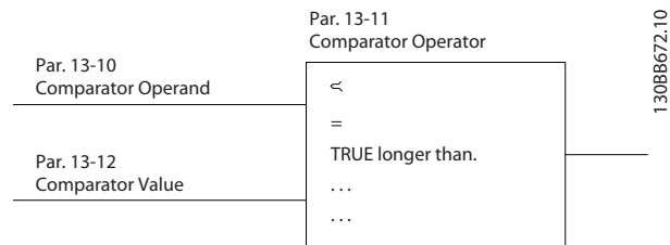
图 4.23 比较器
