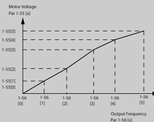
图 4.3 U/f 特性示例
