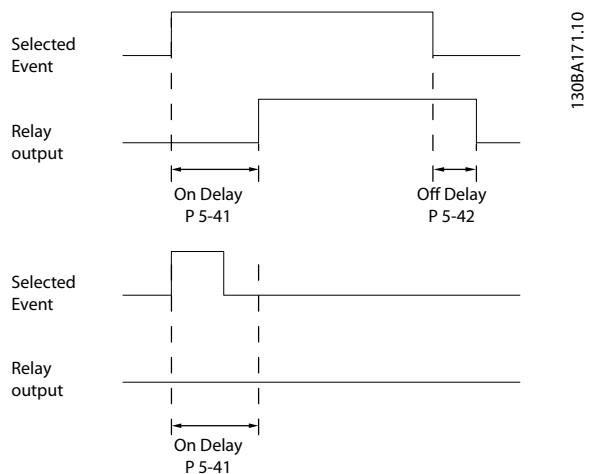
图 4.11 继电器打开延时
