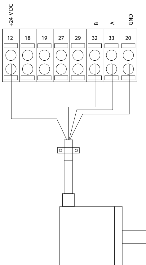
图 4.15 24 V 或 10-30 V 编码器连接
