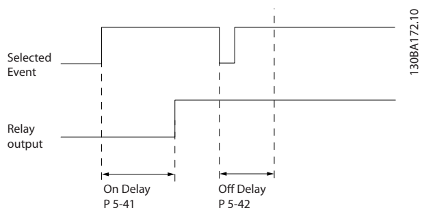
图 4.12 继电器关闭延迟
