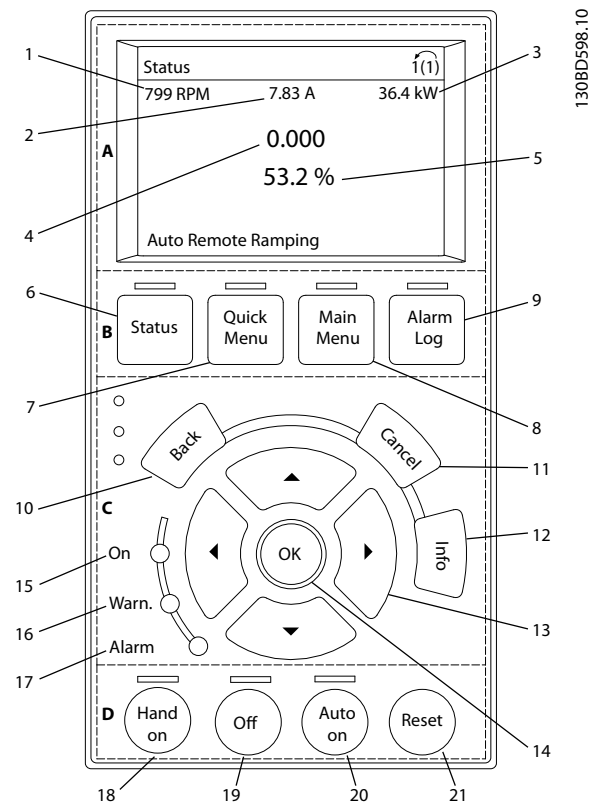
Illustration 5.8 Panneau de commande local graphique (GLCP)
