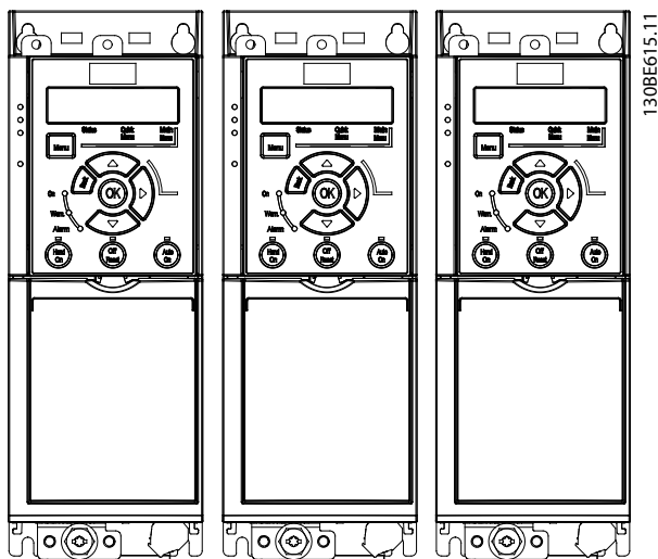
图 3.2 并排安装
