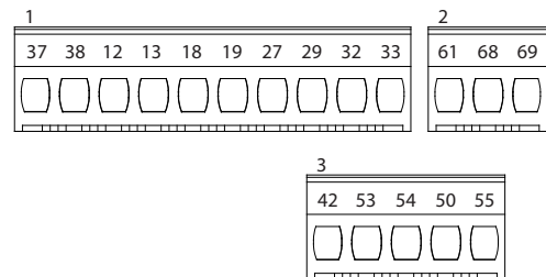
图 4.10 端子号
