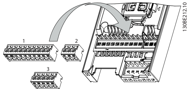
图 4.9 控制端子位置
