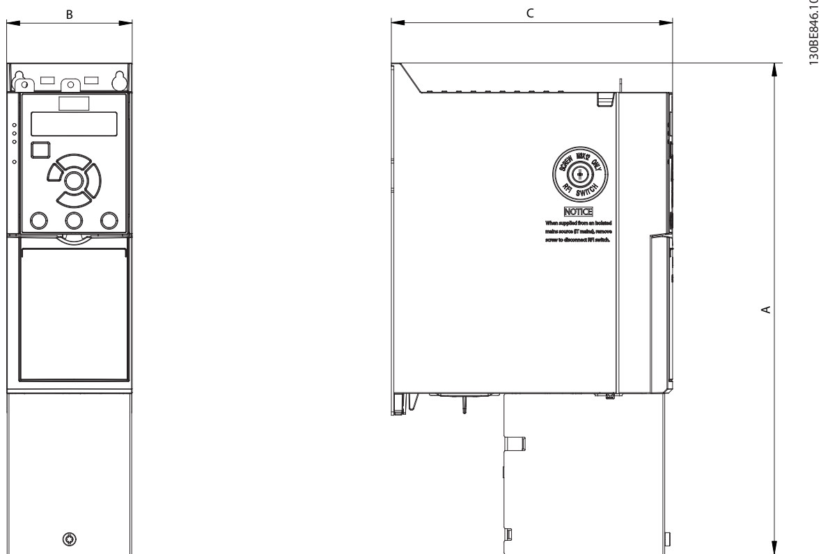
图 9.3 防护等级为 IP21 的标配
