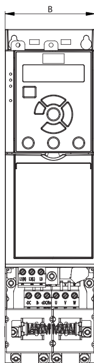
图 9.2 带去耦合板的标配
