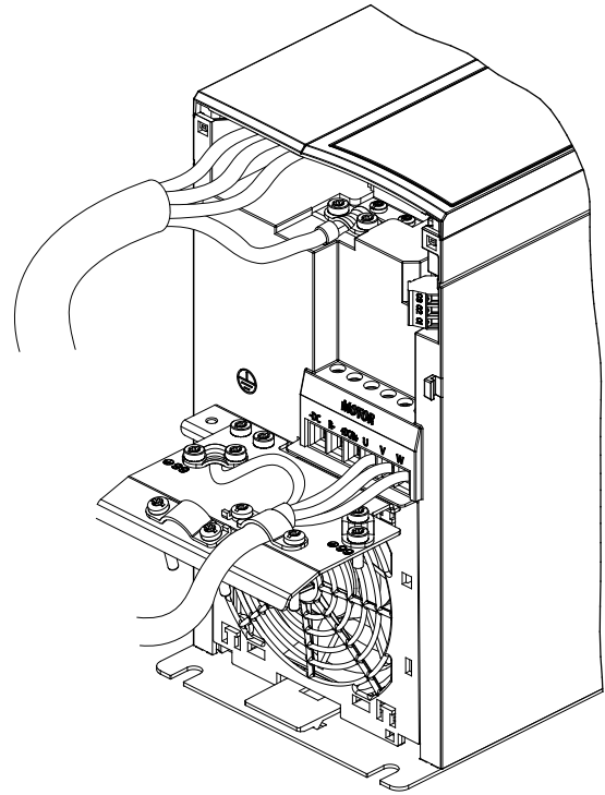
Çizim 4.8 3 fazlı birimler için Şebeke, Motor ve Topraklama bağlantısı (K4, K5)
