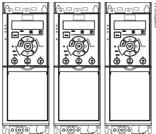
Ilustracja 3.2 Montaż szeregowy
