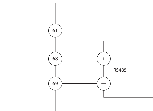
Ilustracja 4.13 Schemat połączeń elektrycznych komunikacji szeregową
