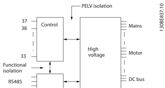
Ilustracja 9.1 Izolacja galwaniczna
