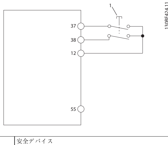
図 6.4 キャビネット 1 個での STO 配線、周波数変換器が電源電圧を供給
