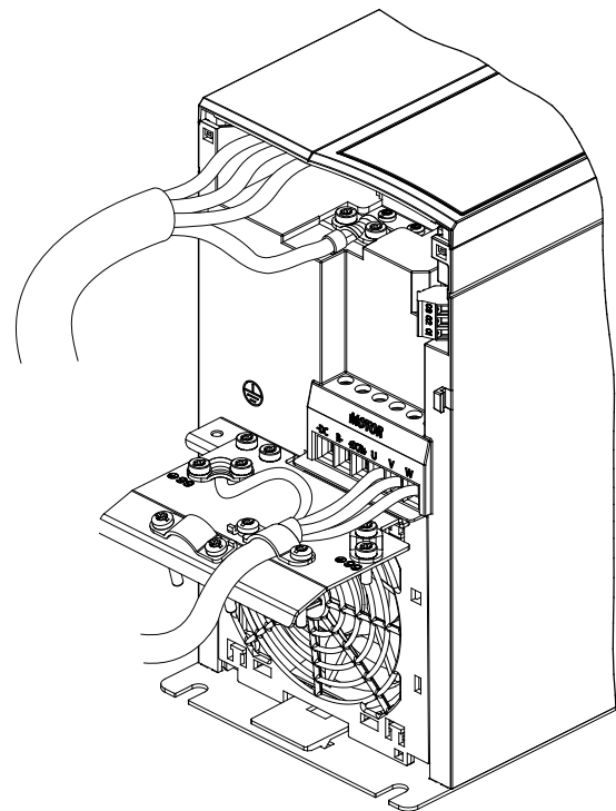
図 4.8 主電源、モーター及び接地接続 (3 相ユニット用) (K4, K5)
