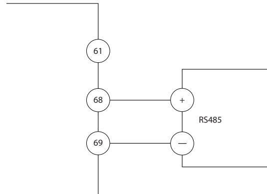
図 4.13 シリアル通信 配線図
