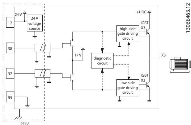
图 6.1 STO 架构
