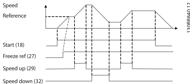
图 7.1 加速/减速
