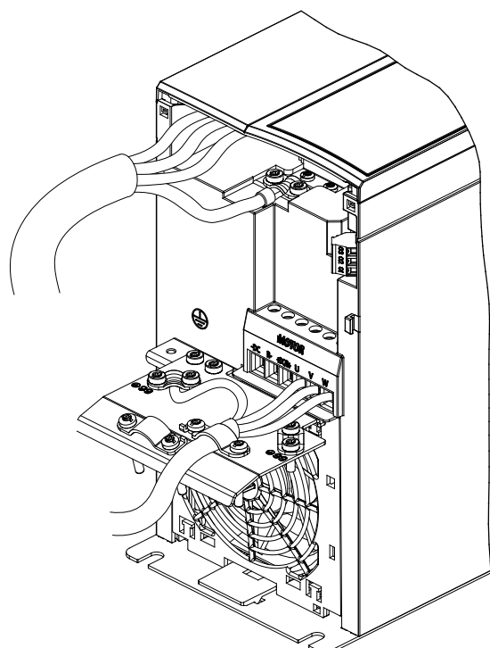
图 4.8 3 相设备的主电源、电机和接地 (K4, K5)
