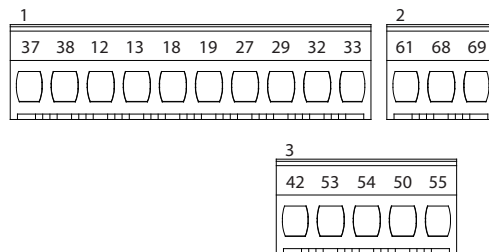
图 4.10 端子号
