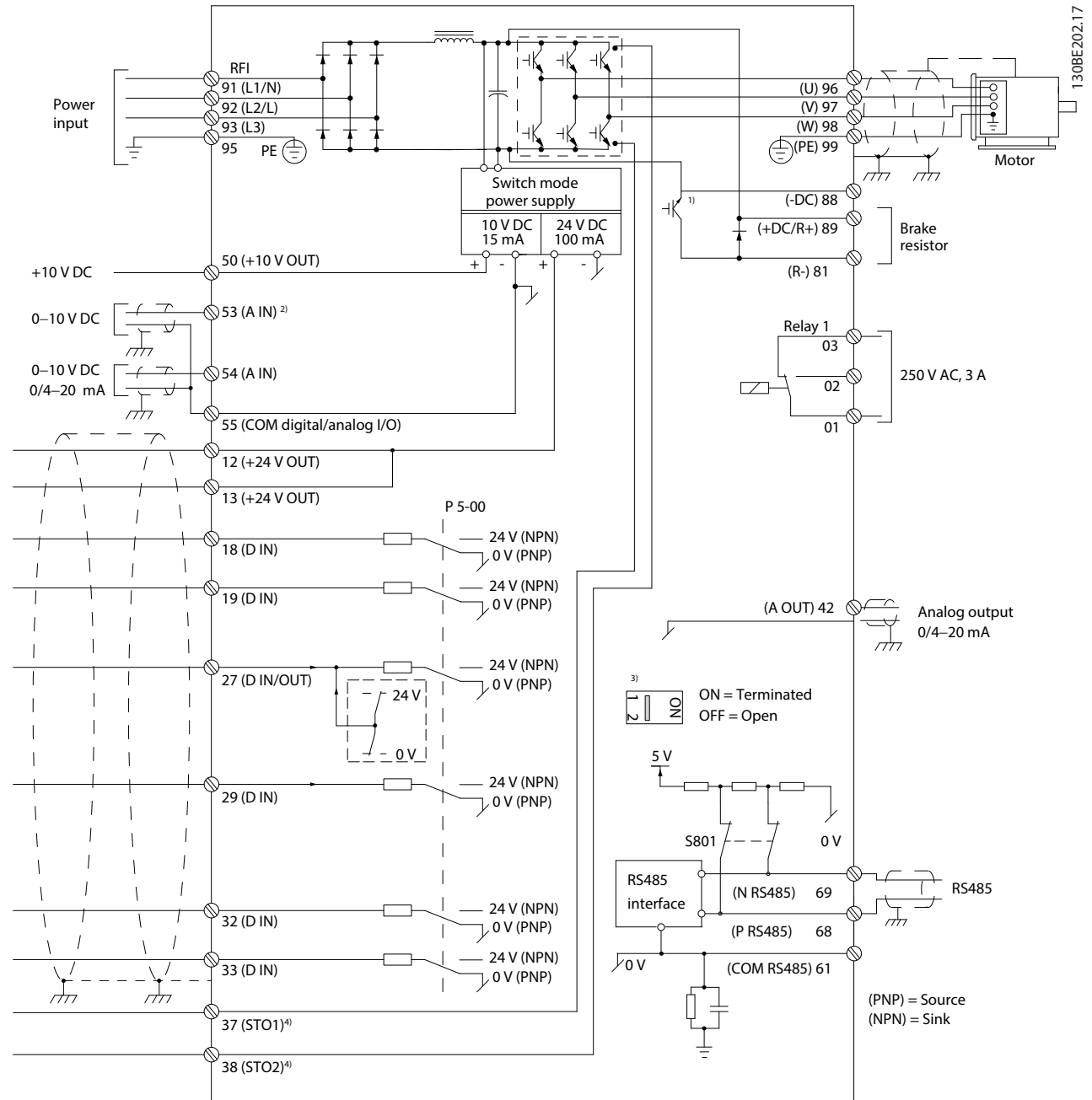
图 4.2 基本接线示意图
