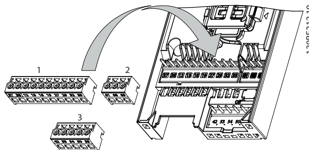
图 4.9 控制端子位置
