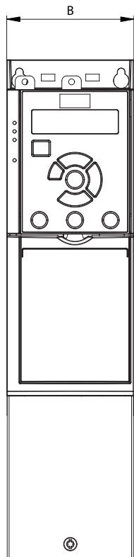
그림 9.3 기본형(하단 케이블 삽입부 덮개 포함(상단 덮개 없음))
