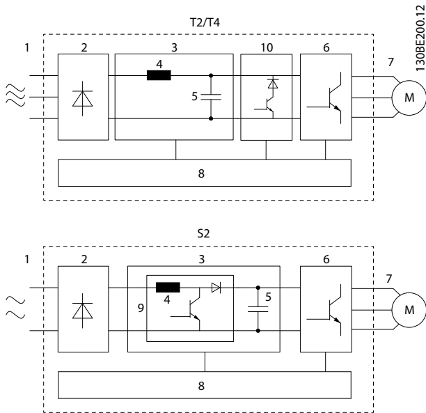
그림 1.1 AC 드라이브의 블록 다이어그램 예시
