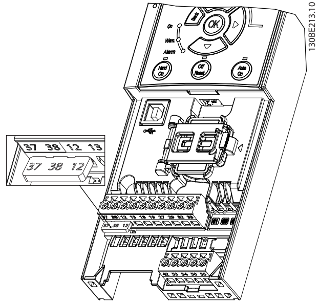
그림 6.3 단자 12 (24 V), 37 및 38 간의 접퍼
