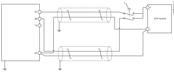
1 안전 장치
