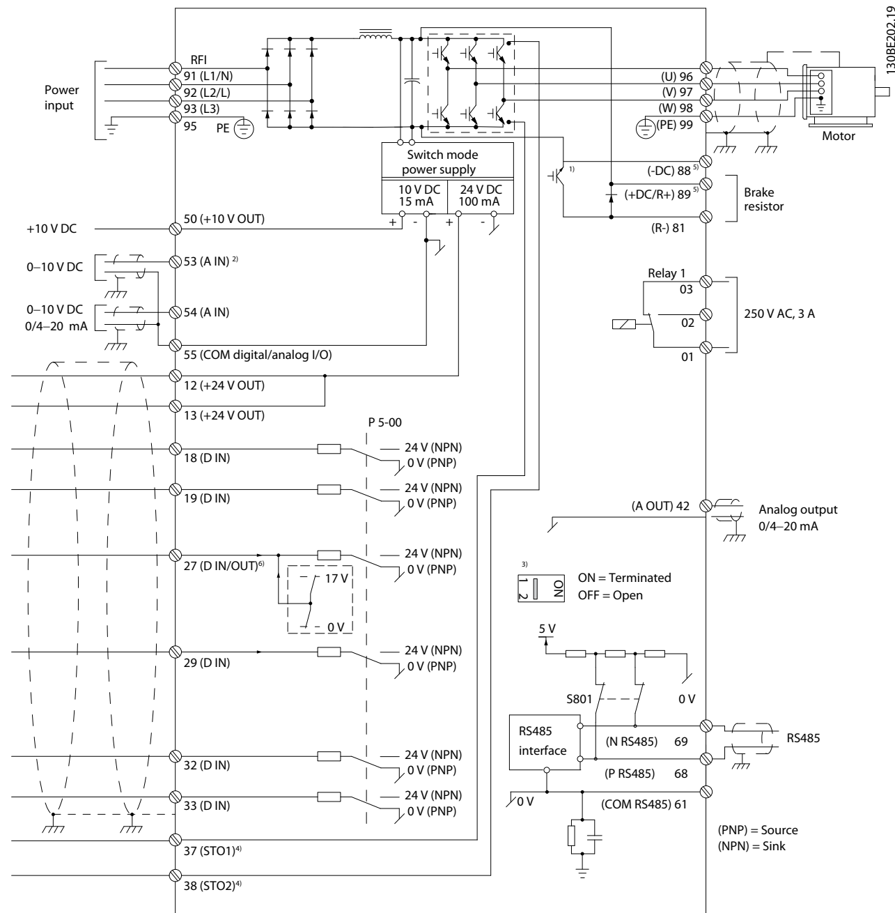
圖 4.2 基本配線概要圖表
