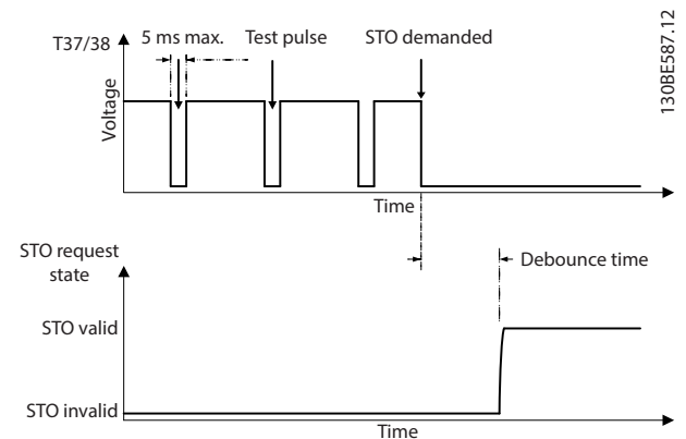
圖 6.2 測試脈衝濾波
